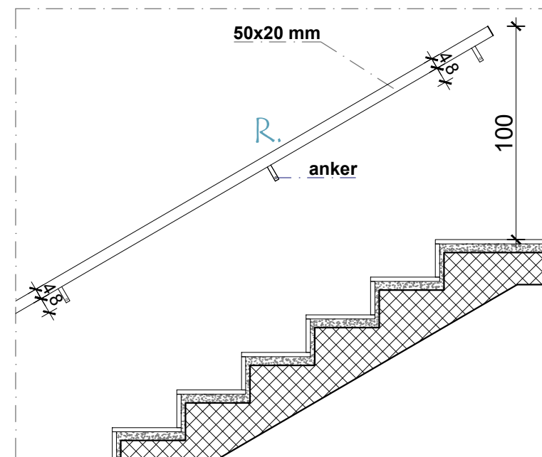
izgled
