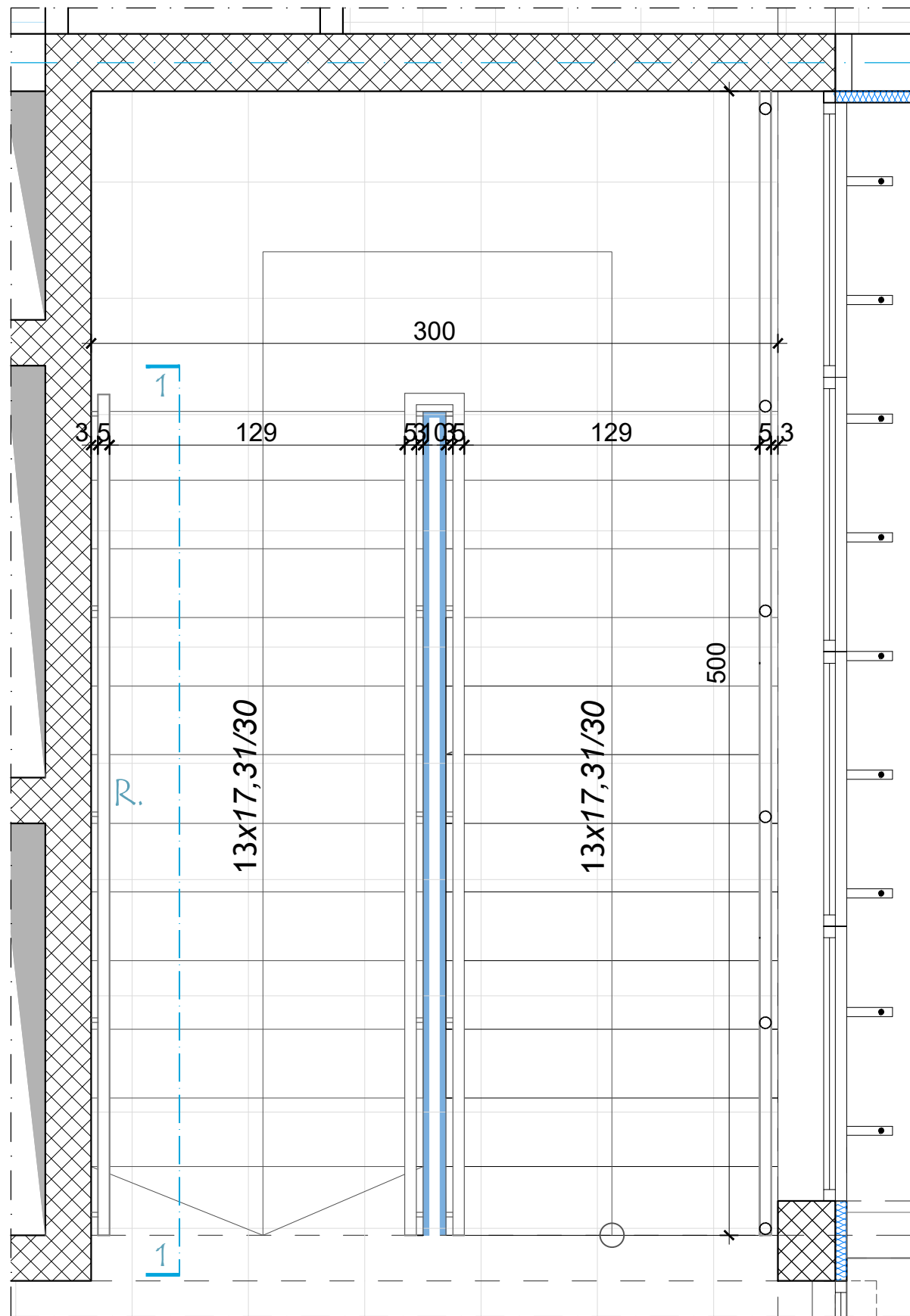
Rukohvat "R" osnova
