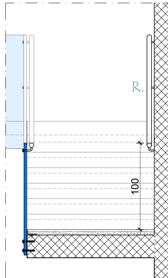
presjek "1-1"
