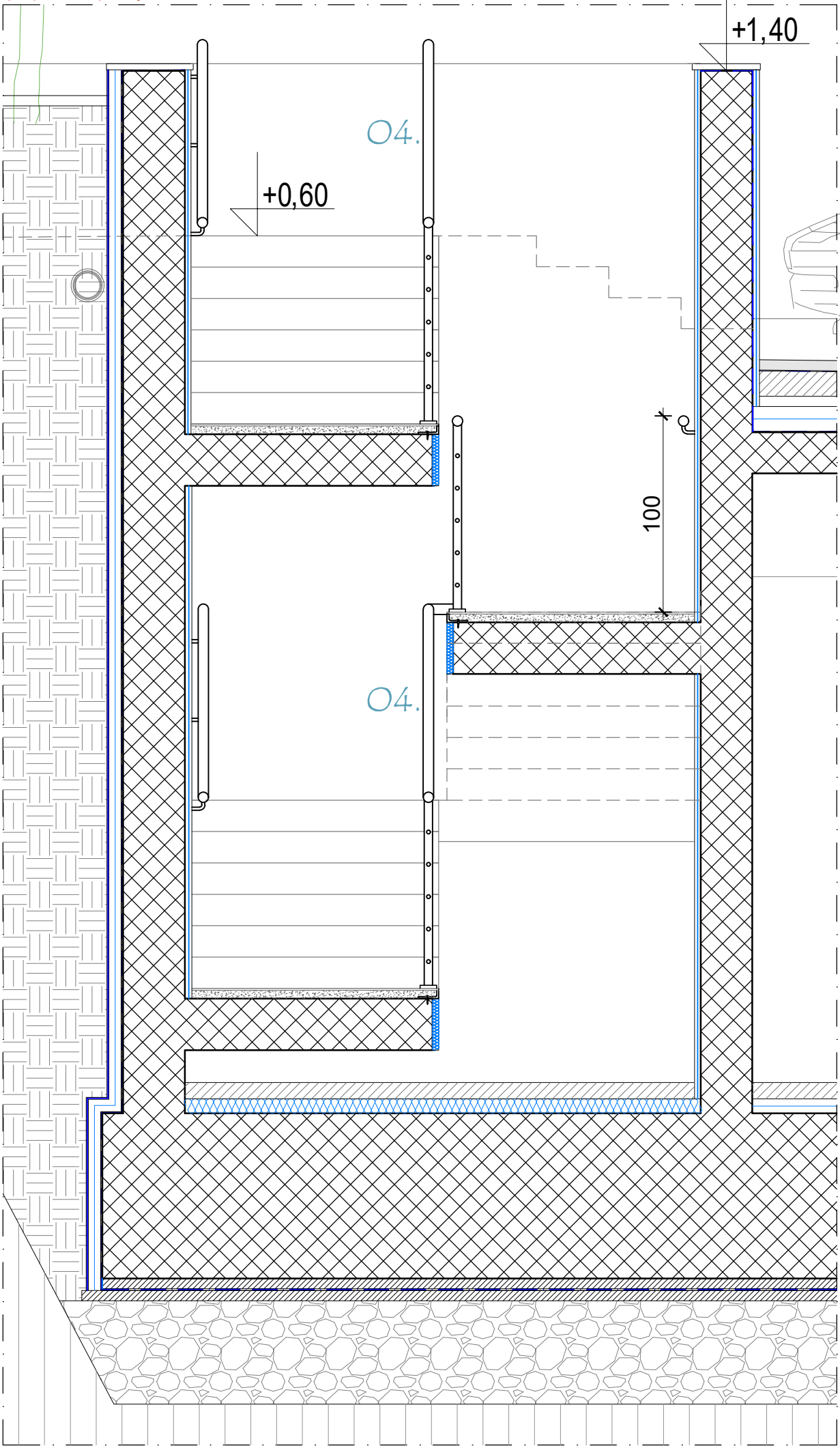
poprečni presjek
