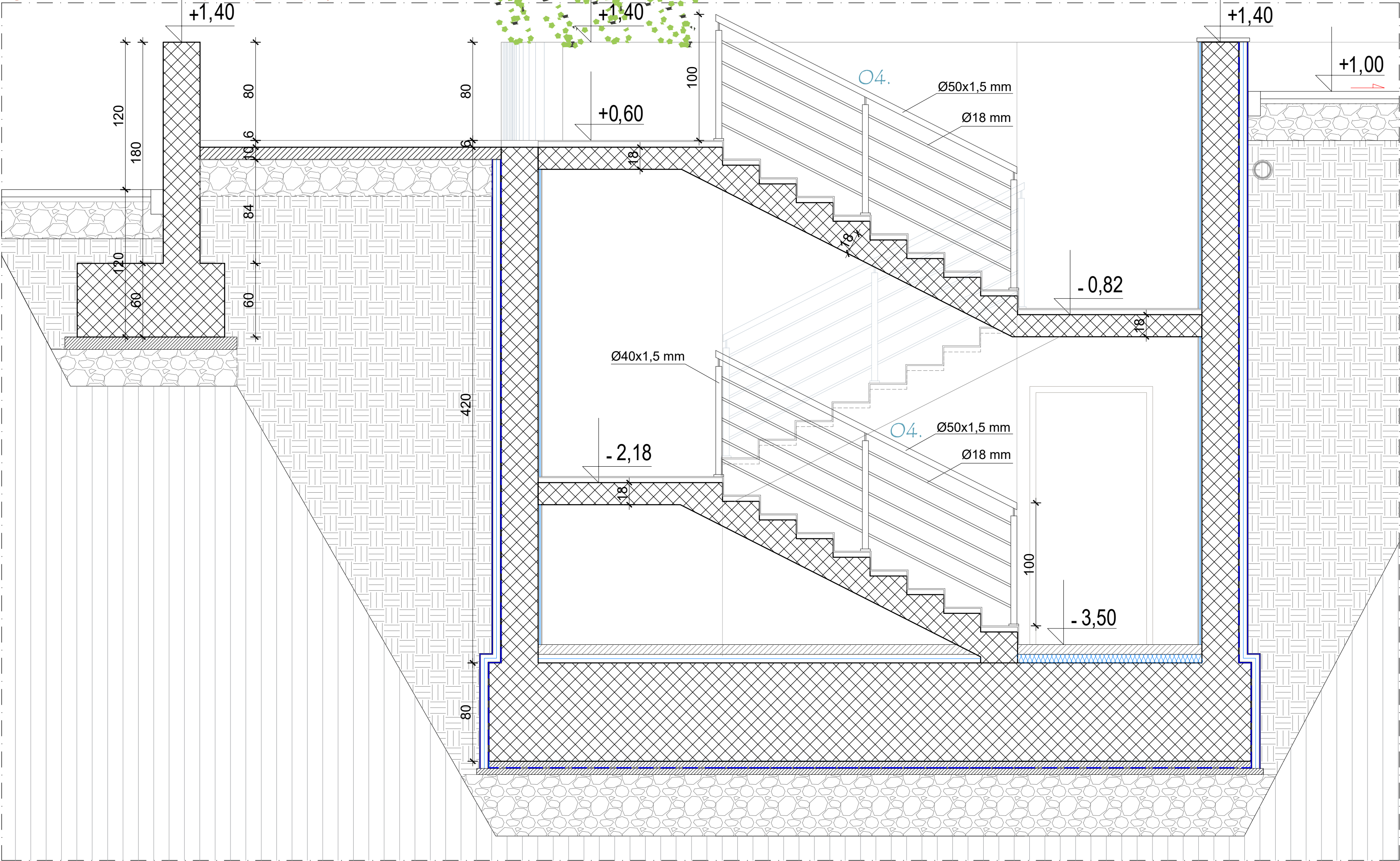
Ograda "O2" na evakuacionom stepeništu _podužni presjek
