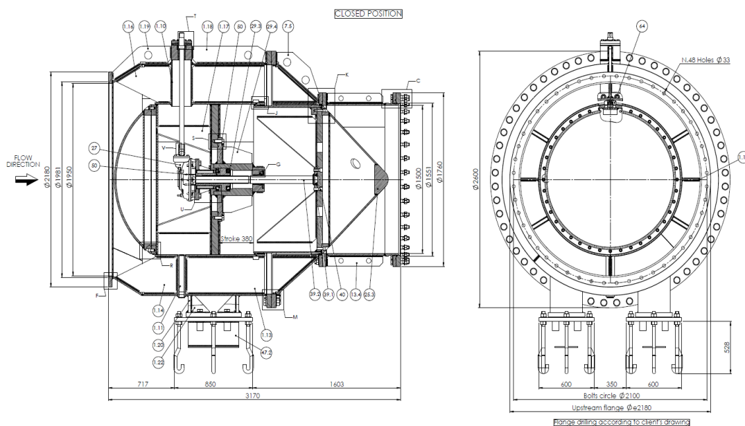
Slika 1: Džonsonov igličasti zatvarač
