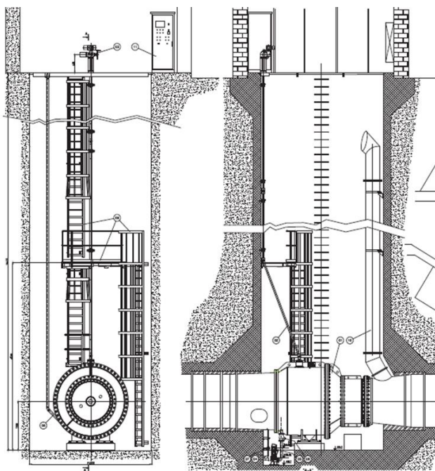
Slika 2: Pozicija igličastog zatvarača u jami
