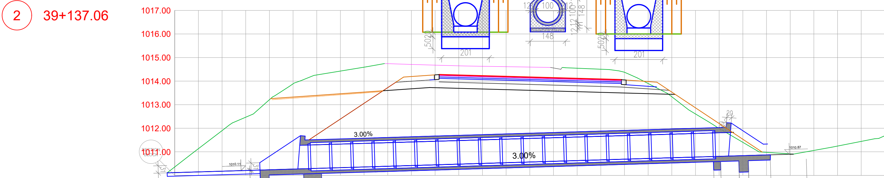
Cjevasti proput Ø1000 Sta: 39+137.06
