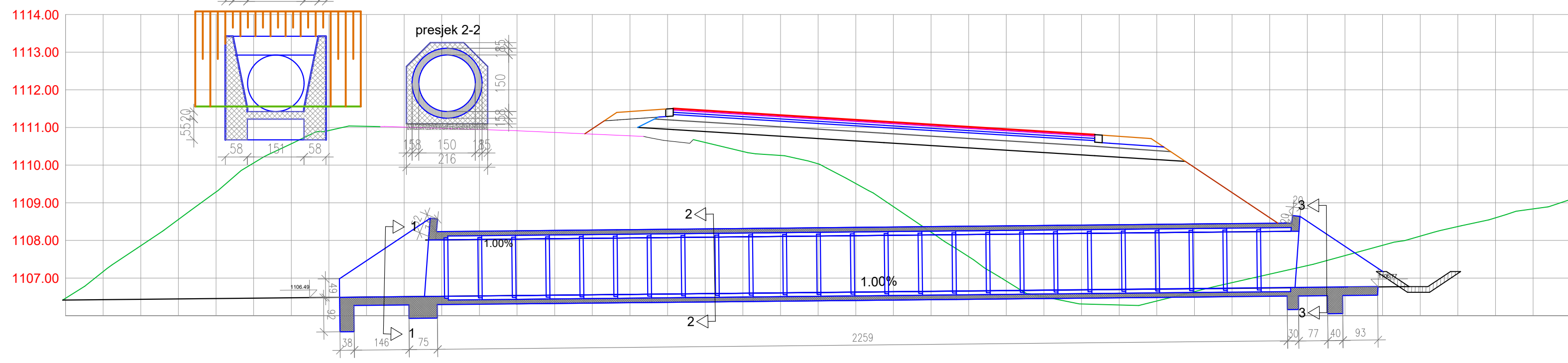
Cjevasti proput Ø1500 Sta: 44+124.03
