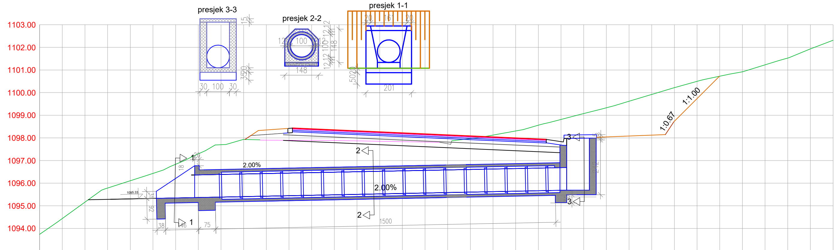
Cjevasti proput Ø1000 Sta: 43+880.94
