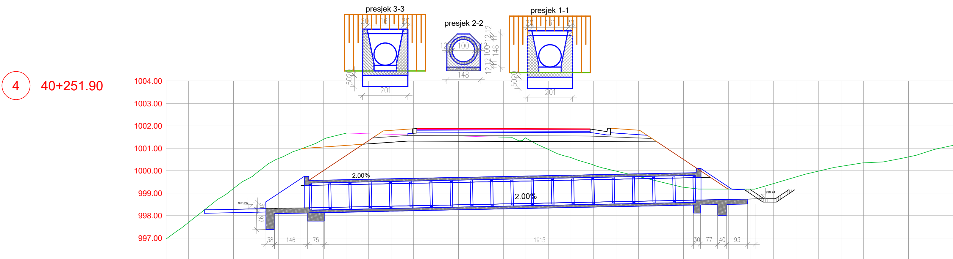
Cjevasti proput Ø1000 Sta: 40+251.90
