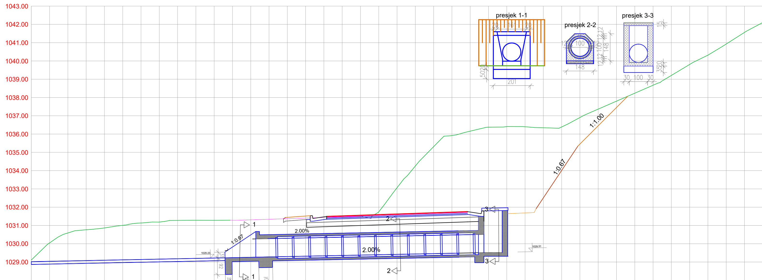
Cjevasti proput Ø1000 Sta: 42+102.76
