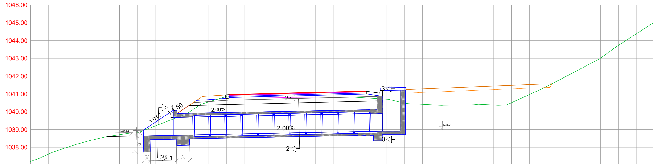
Cjevasti proput Ø1000 Sta: 42+484.23
