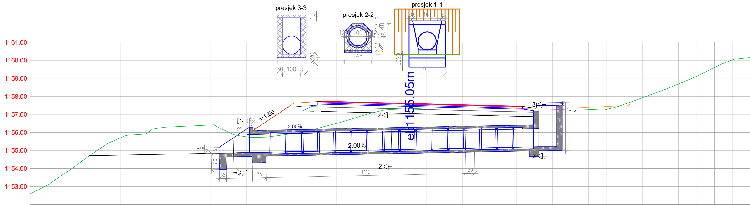
Cjevasti proput Ø1000 Sta: 45+136.21
