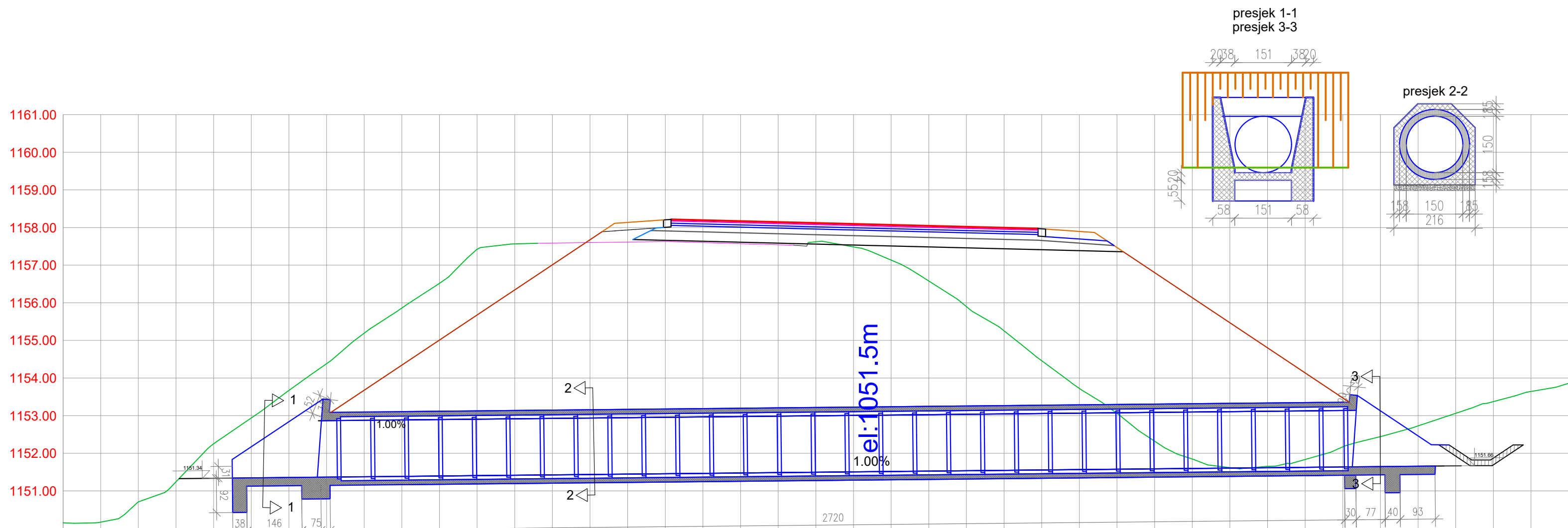
Cjevasti proput Ø1500 Sta: 45+584.78
