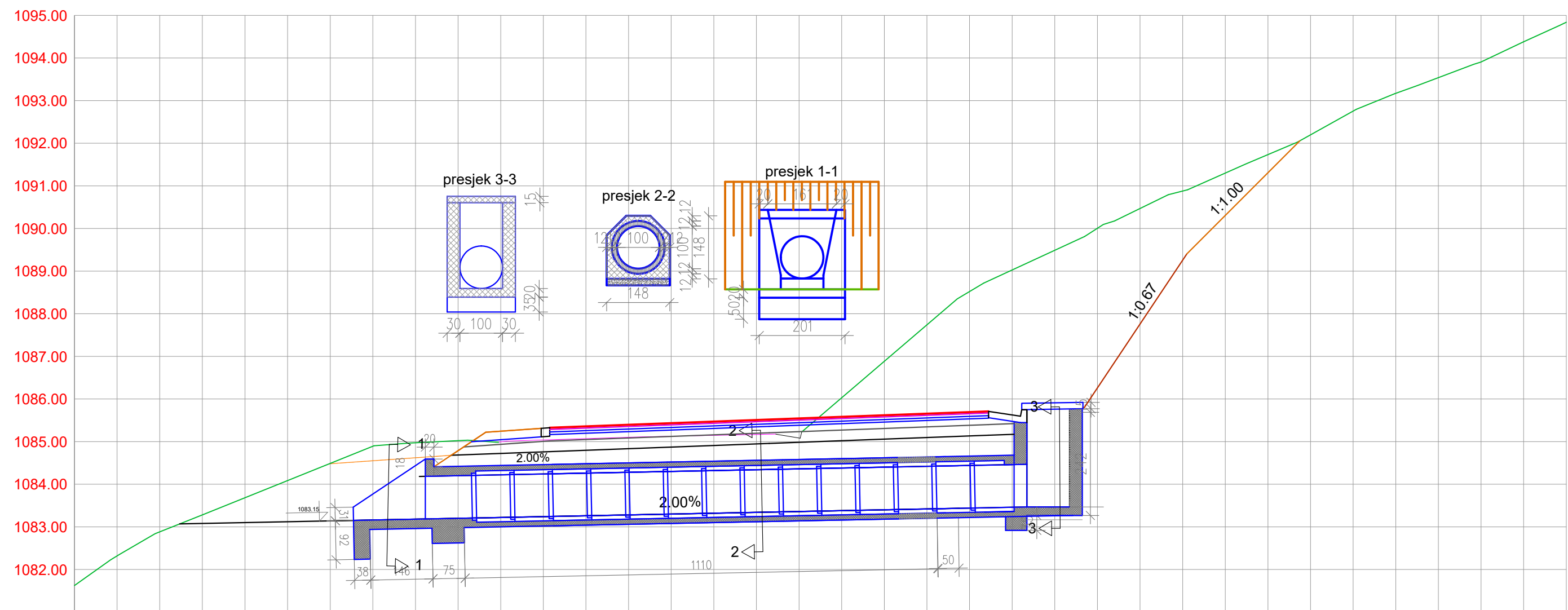
Cjevasti proput Ø1000 Sta: 43+641.86
