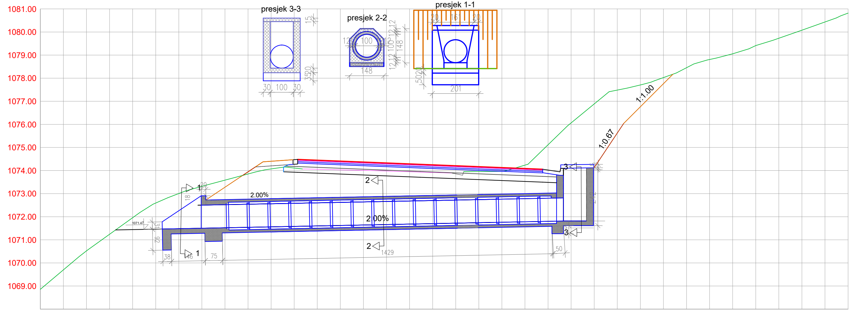
Cjevasti proput Ø1000 Sta: 43+433.63
