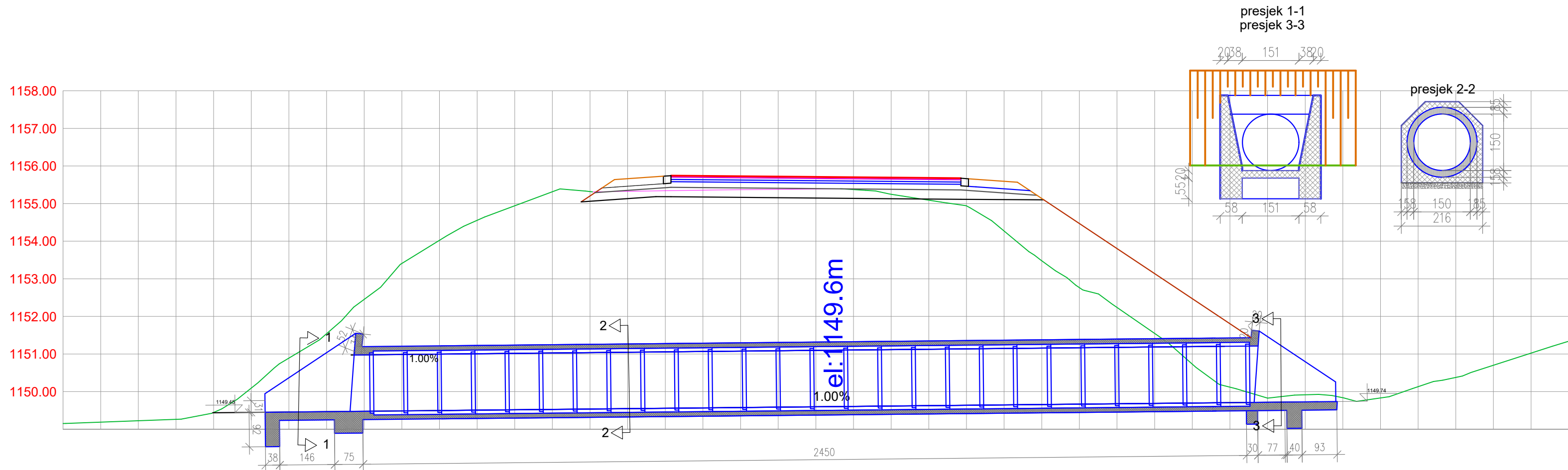
Cjevasti proput Ø1500 Sta: 45+700.00
