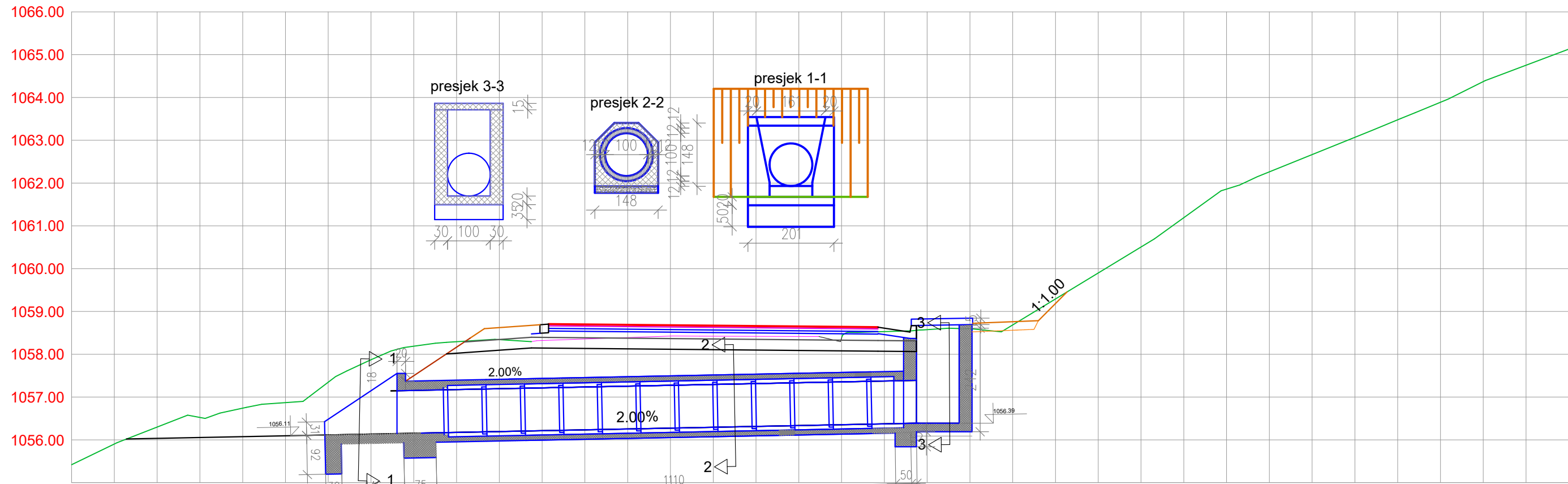
Cjevasti proput Ø1000 Sta: 43+122.74
