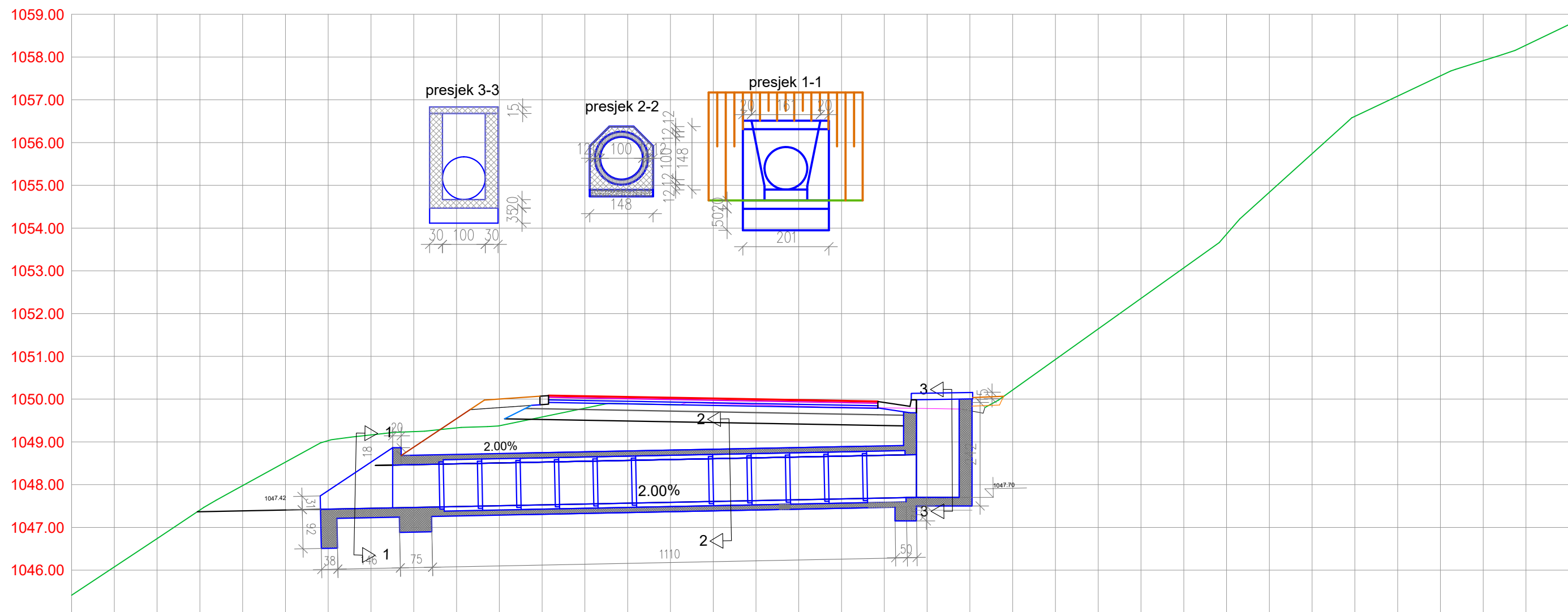
Cjevasti proput Ø1000 Sta: 42+846.62
