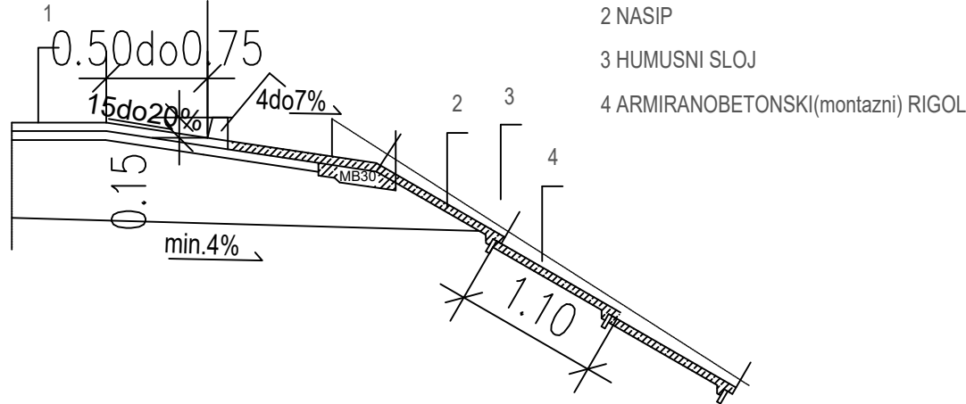
Presjek A-A
