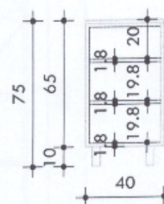
BOČNI IZGLED
