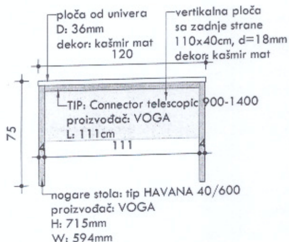
FRONTALNI IZGLED
