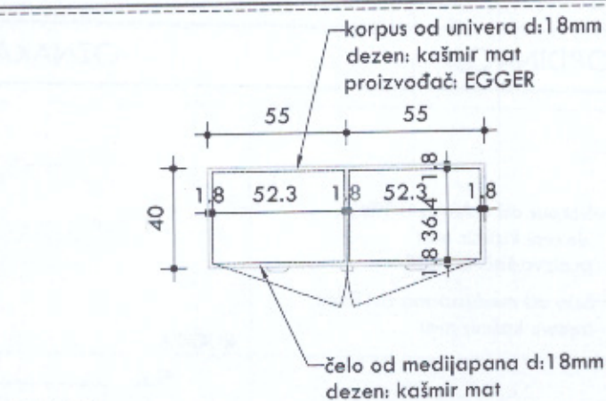
OSNOVA
