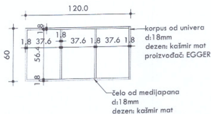
OSNOVA
