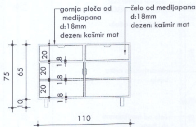
FRONTALNI IZGLED
