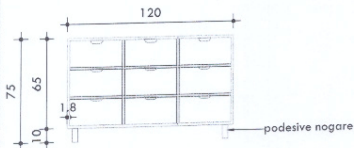
FRONTALNI IZGLED
