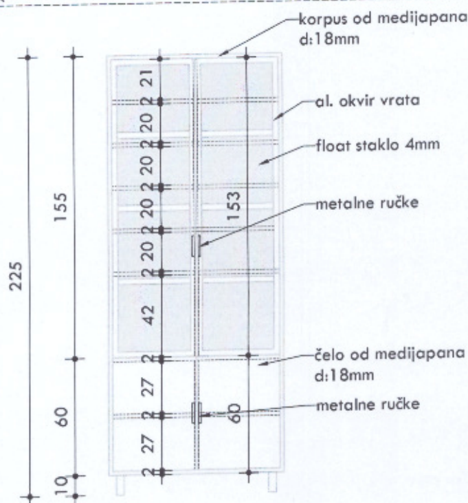
FRONTALNI IZGLED
