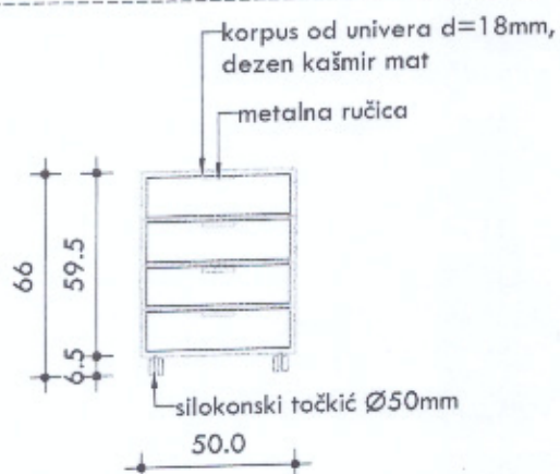
FRONTALNI IZGLED
