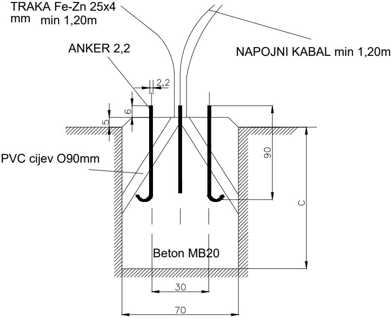
SKICA TEMELJA SA RASPOREDOM ANKERA
