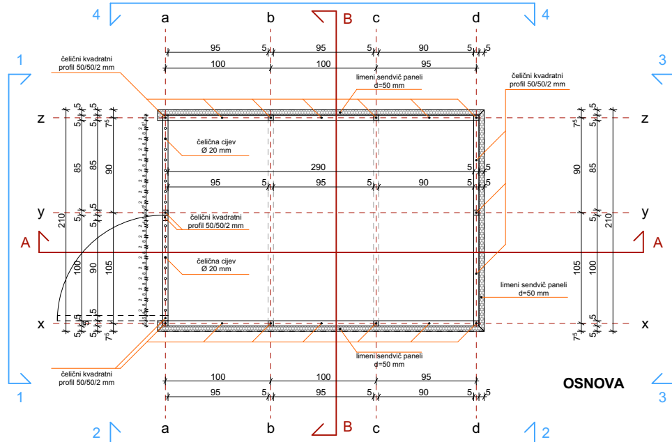
OSNOVA KROVA
