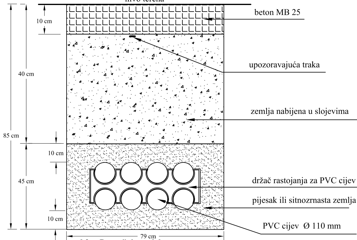
sl.2 – Poprečni presjek rova u trotoaru
