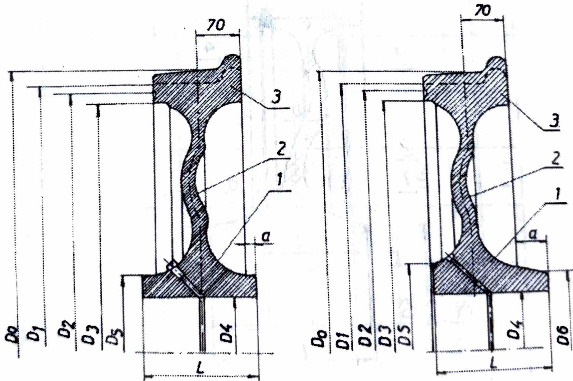
Slika 6. Monoblok točkovi: 1-glavčina, 2-ploča, 3-obod
