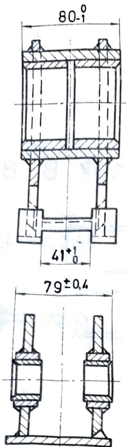
Zavarena konstrukcija
