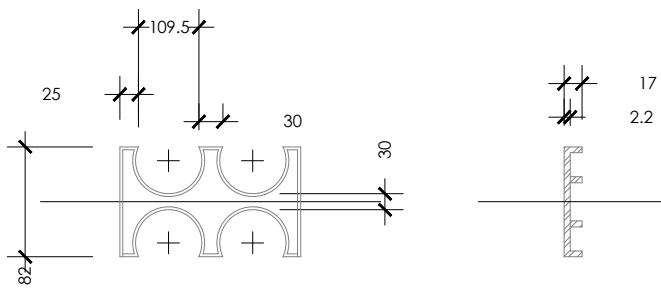
sl. 3 -- Držać rastojanja za 4 cijevi Ø110 mm (110/4)
