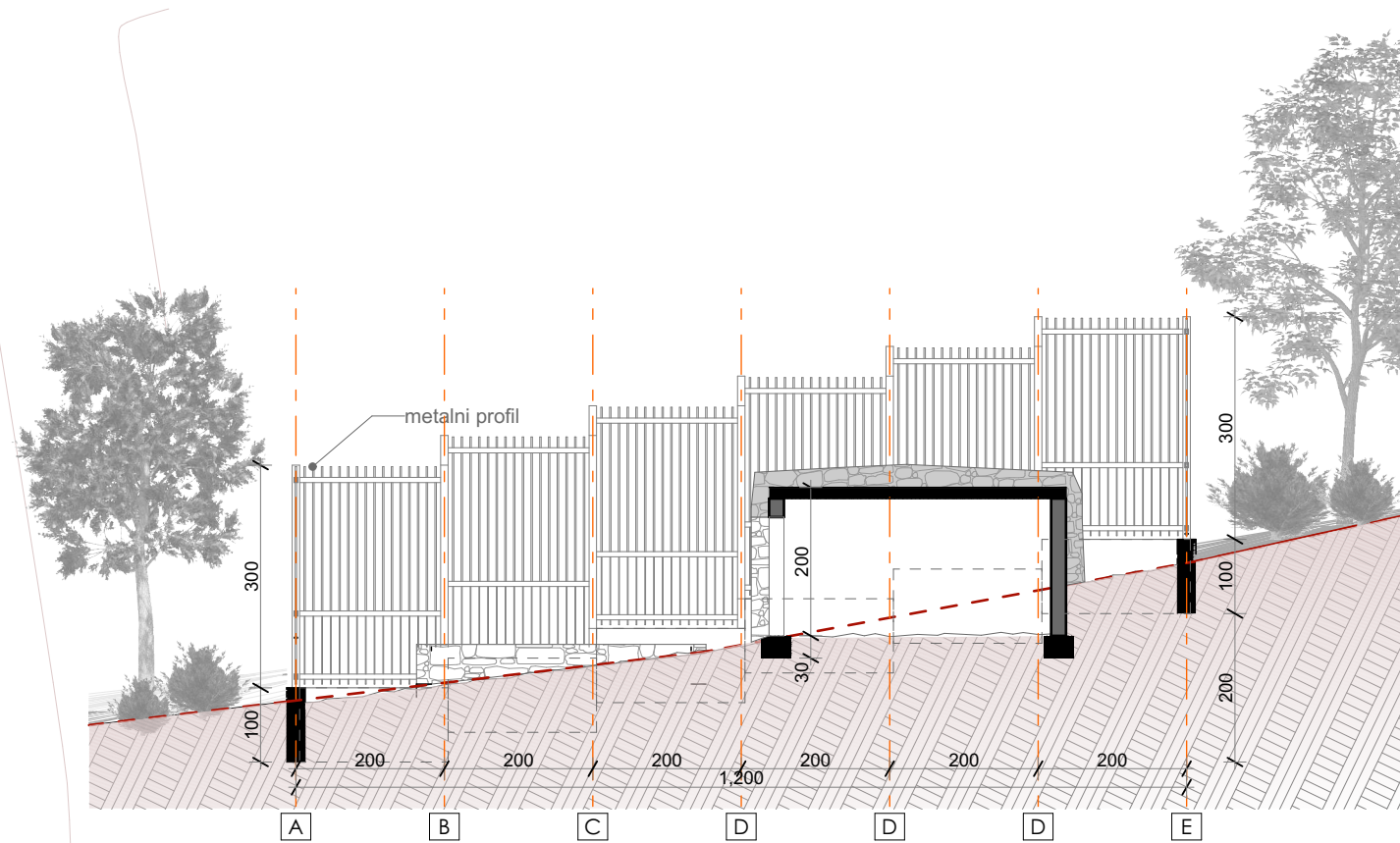
PRESJEK 1-1
