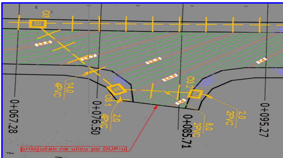
Slika 2: Na početku zahvata detalj infrastrukture iz glavnog projekta "Ulica "2" po DUP-u "Ilino" u Baru".
