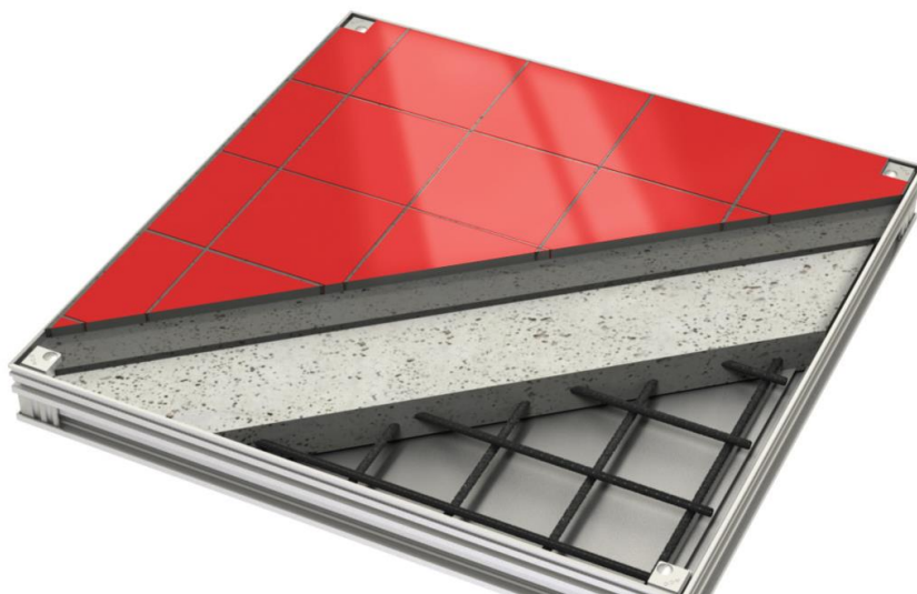
Slika 23: Izgled strukture ambijentalnog pokopca
