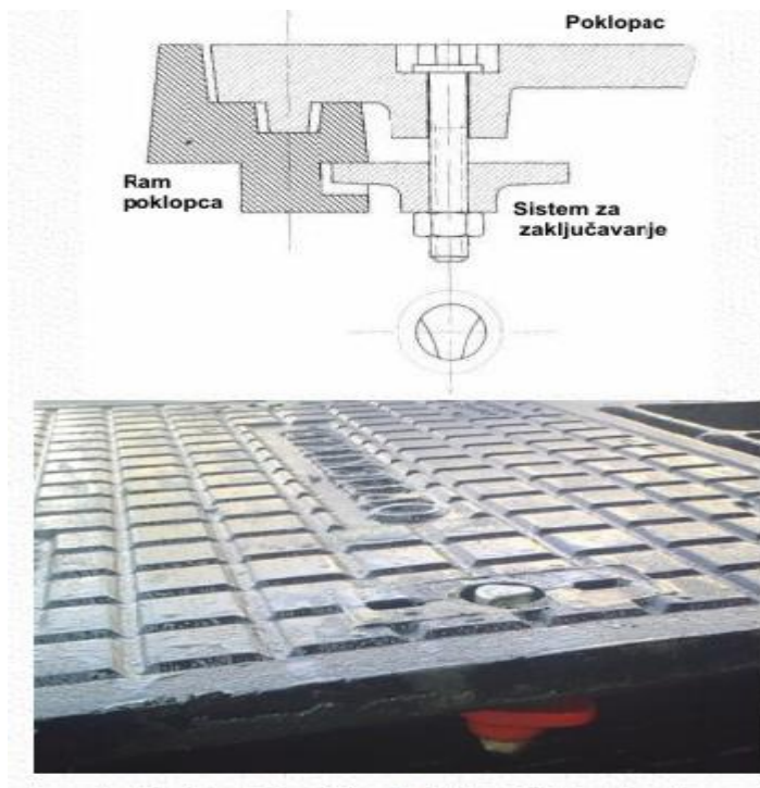
Slika 8: Sistem za zaštitu od krađe
