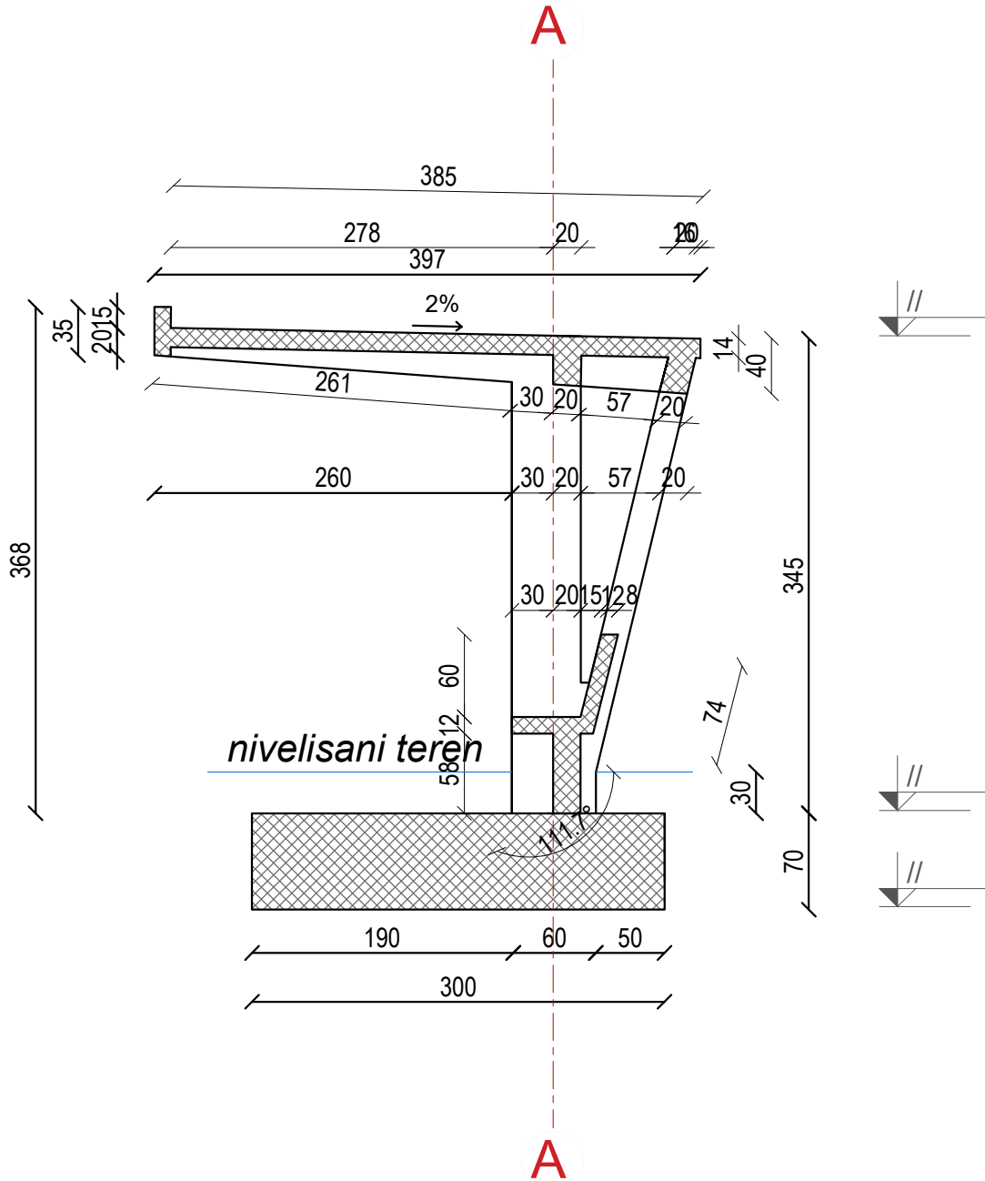
Poprečni presjek 2-2
