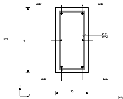
Presek 37-37 x = 4.32m
