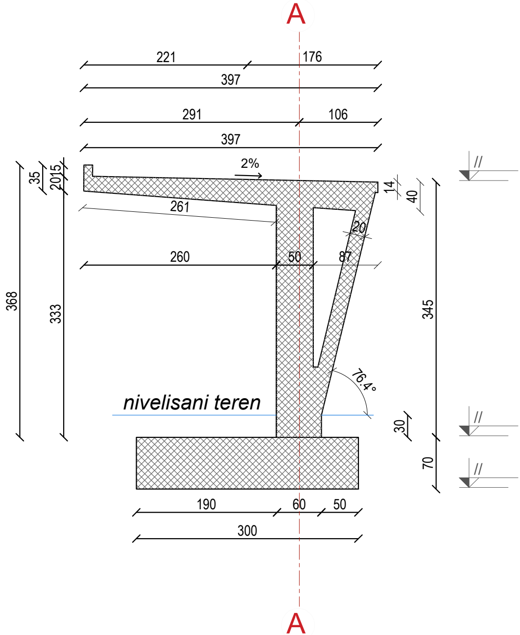
Poprečni presjek 1-1
