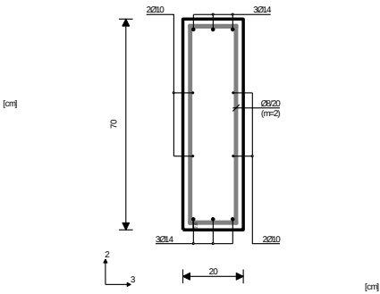
Presek 6-6 x = 4.23m
