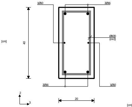
Presek 33-33 x = 4.32m
