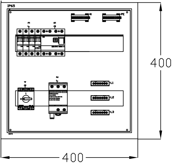
Ormar RO-AC-PV-S2
