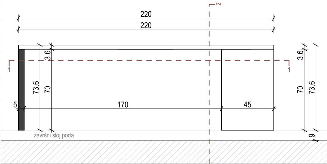
RADNI STO_presjek 1
