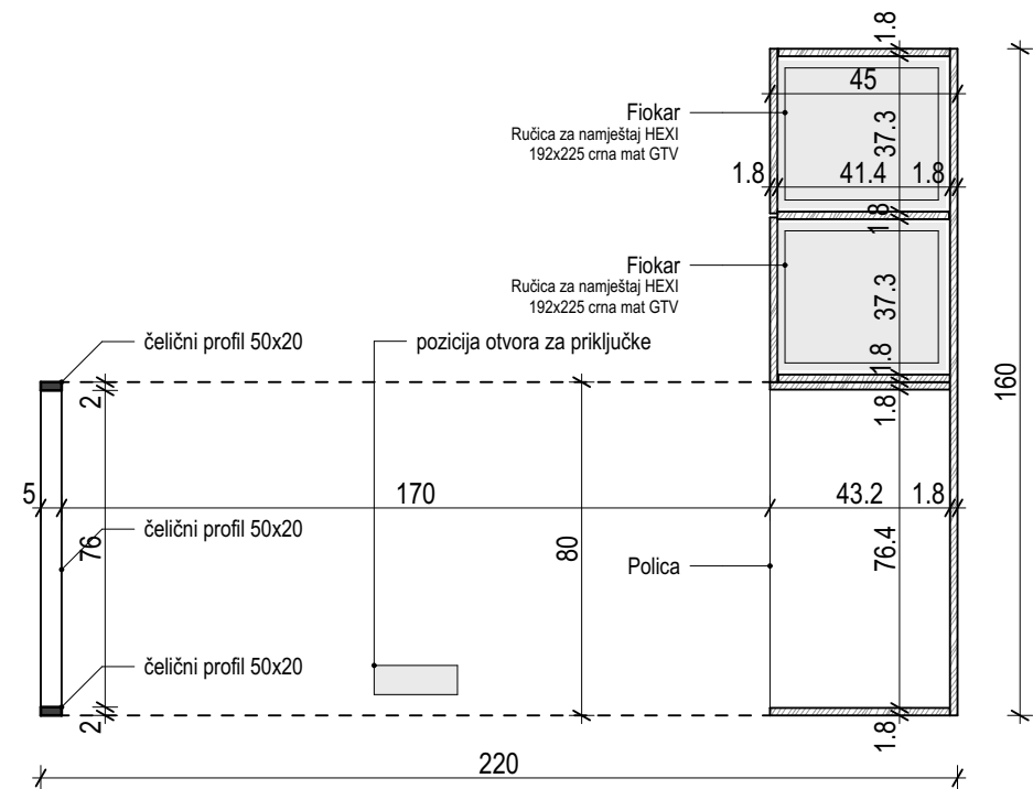
RADNI STO_presjek 2
