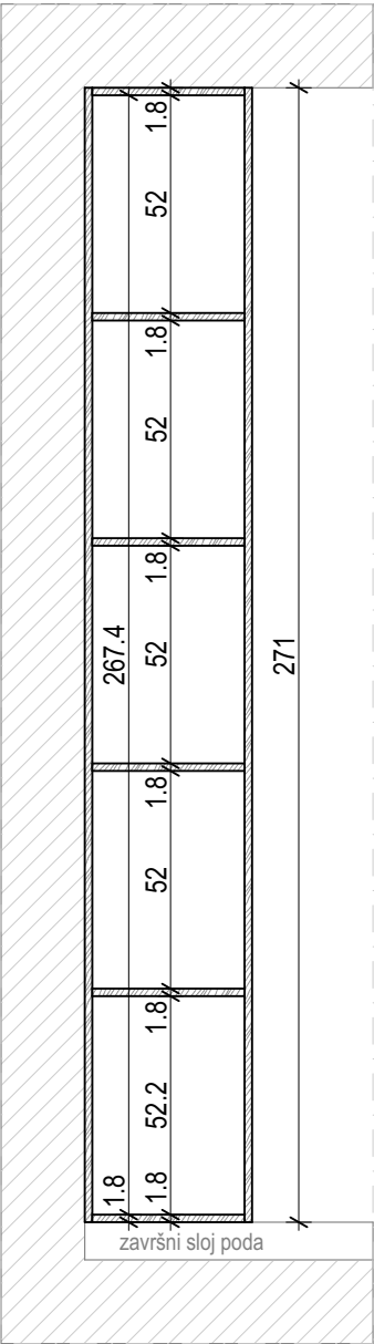
ORMAR_presjek 2
