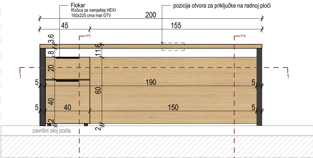
RADNI STO_presjek 1
