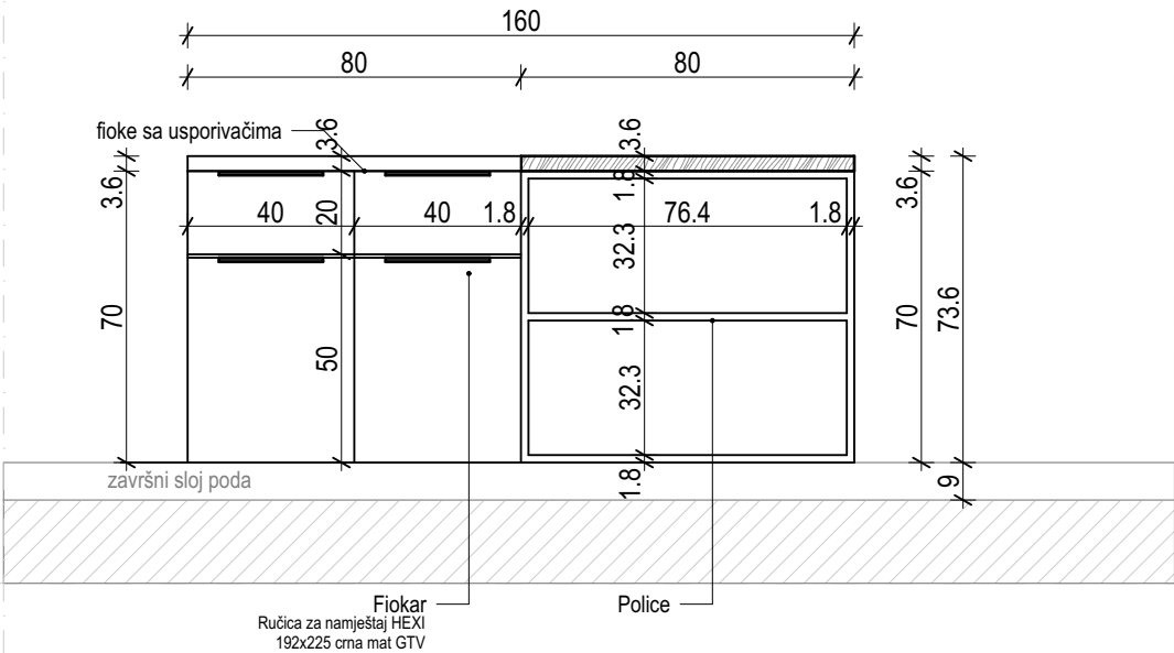
RADNI STO_presjek 2
