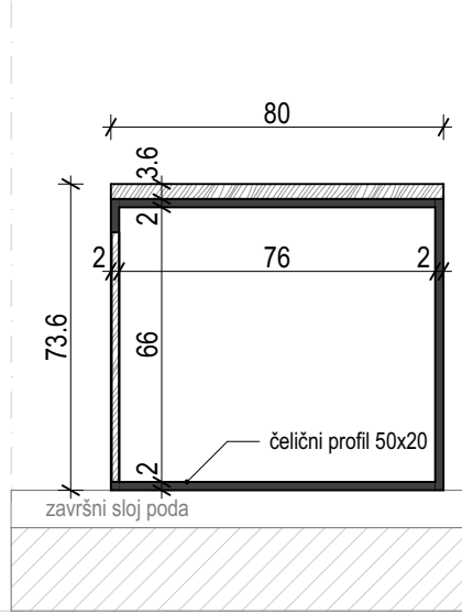
RADNI STO_presjek 3
