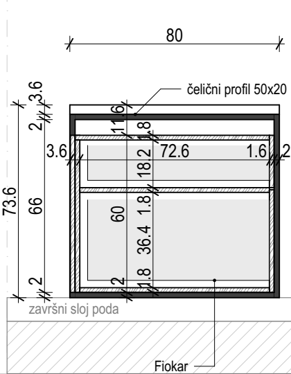
RADNI STO_presjek 3
