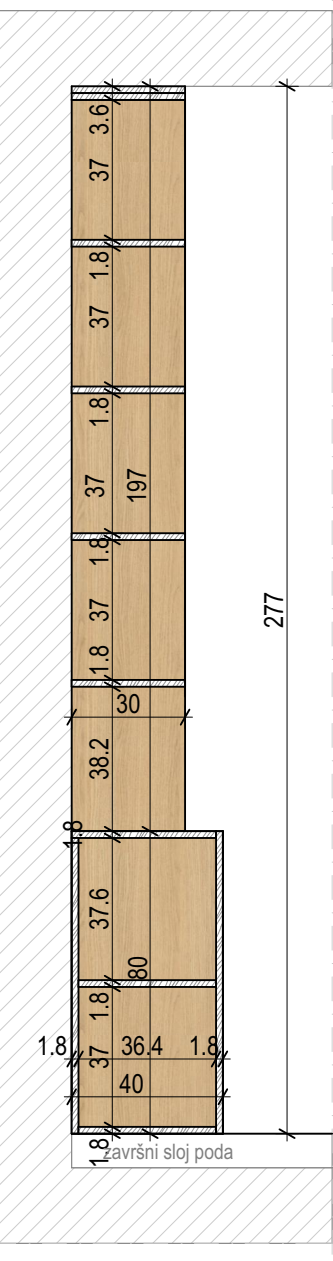
POLICA_presjek 3
