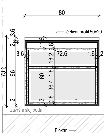
RADNI STO_presjek 3
