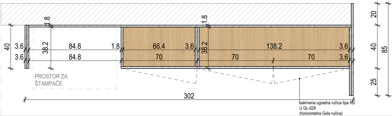
POLICA_presjek 2
