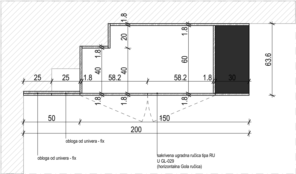
ORMAR_presjek 1
