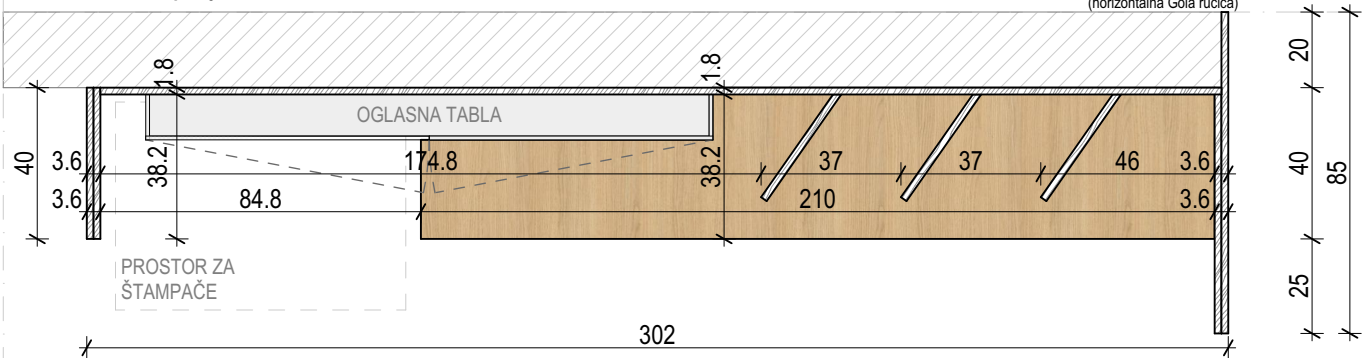
POLICA_presjek 1
