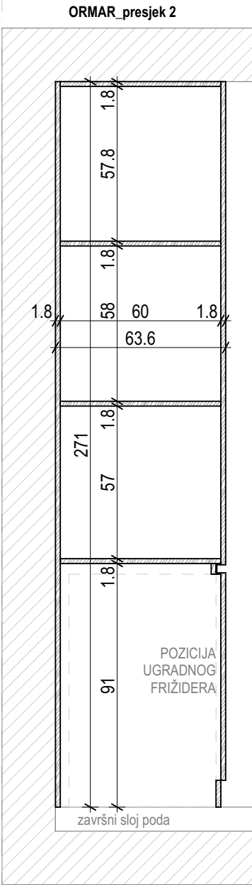
ORMAR_presjek 2
