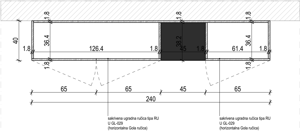
ORMAR_presjek 1
