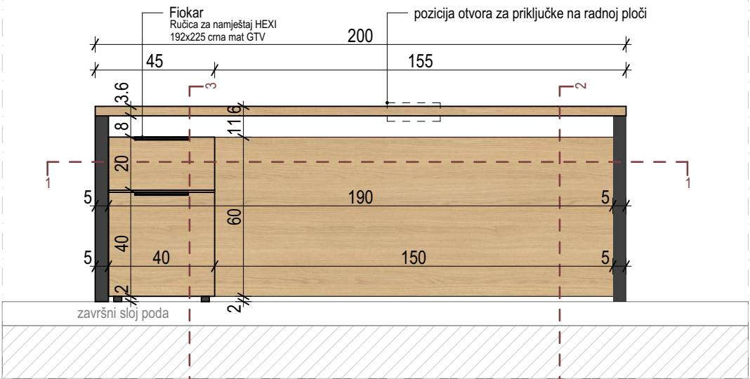
RADNI STO_presjek 1
