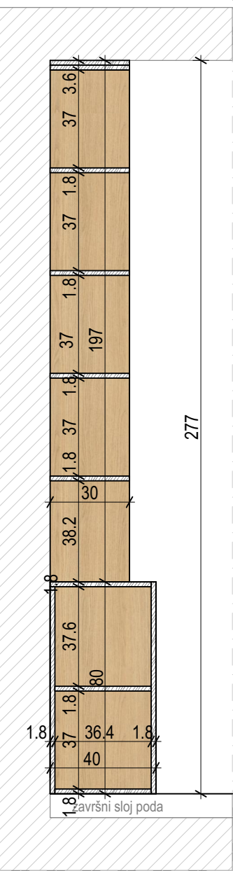
POLICA_presjek 3
