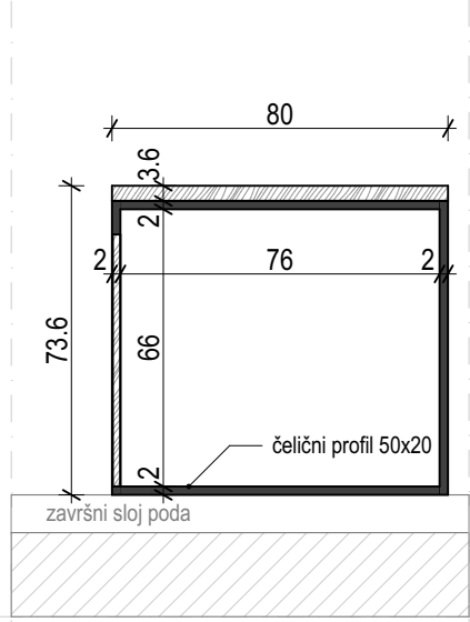
RADNI STO_presjek 3
