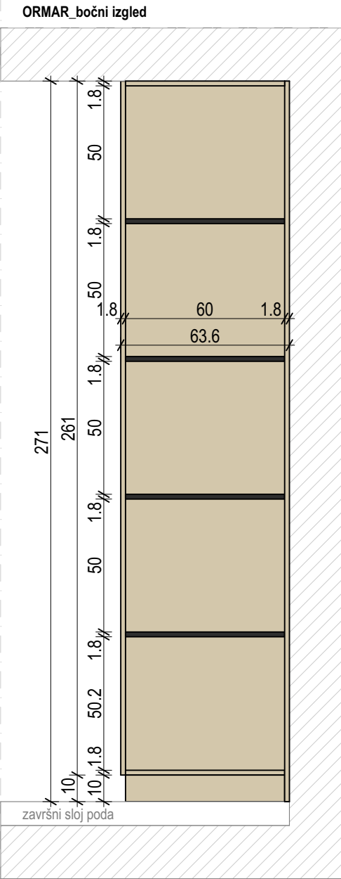
ORMAR_bočni izgled
