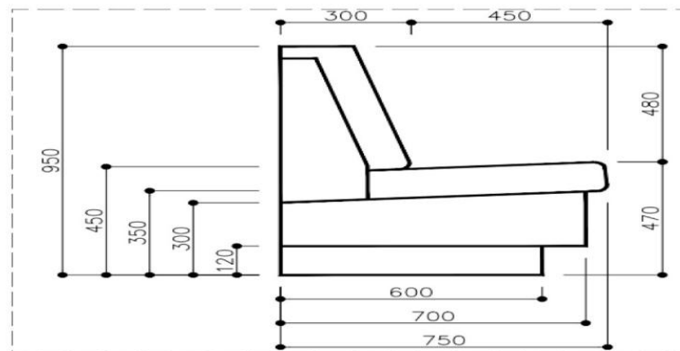
presjek sofe
