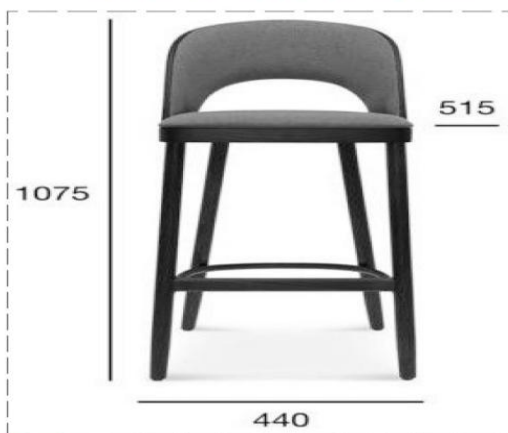
tehnička skica barske stolice
