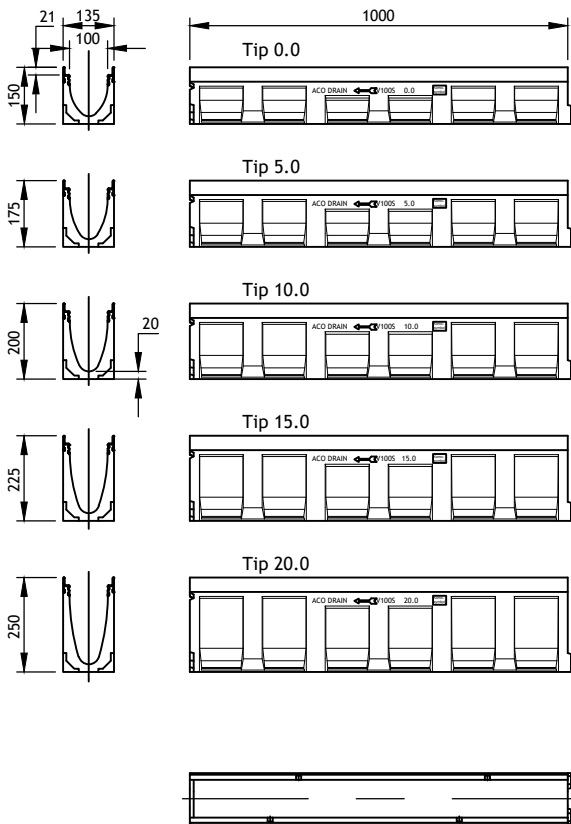
ACO Multiline V100 1m
