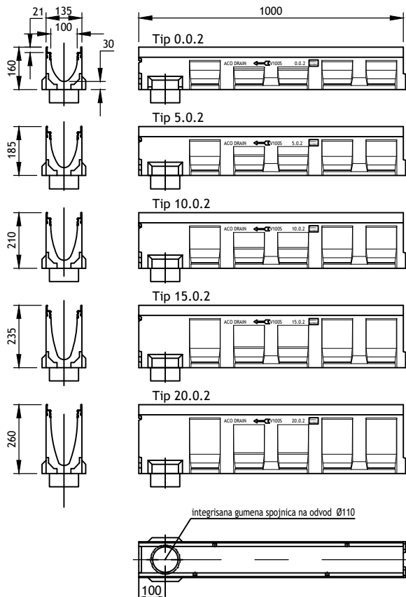
ACO Multiline V100 1 m sa integrisanom gumenom spojnicom na odvod Ø110
