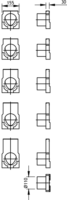
Čeoni poklopac sa priključkom Ø110
