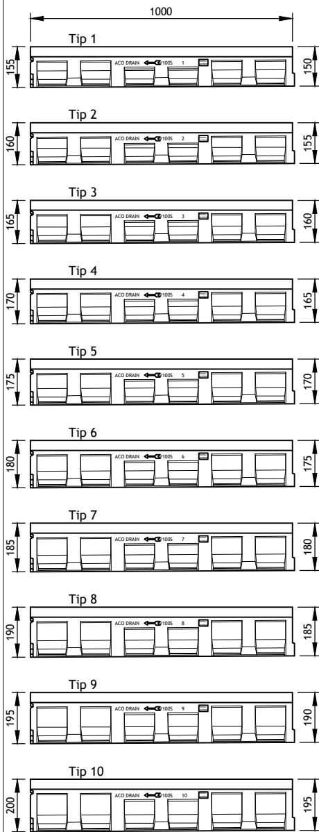
ACO Multiline V100 1m, pad dna i=0,5%
