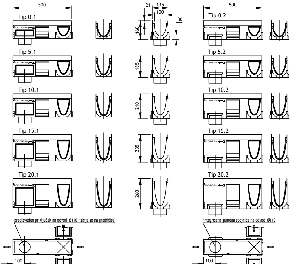
ACO Multiline V100 0,5 m sa mogućim spojevima kanala u obliku L ili T i integrisanom gumenom spojnicom na odvod Ø110
