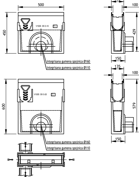
Sabirno okno sa bočnim priključkom
