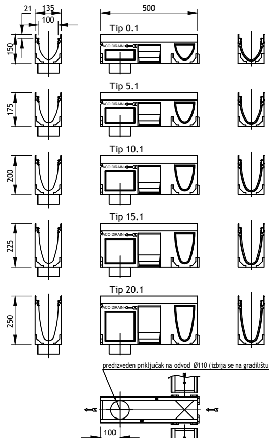
ACO Multiline V100 0,5 m sa mogućim spojevima kanala u obliku L ili T i predizvedenim priključkom na odvod Ø110
