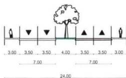
Tip 3 - SAOBRAĆAJNICE III REDA
