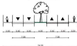
Tip 2: SAOBRAĆAJNICE I REDA
