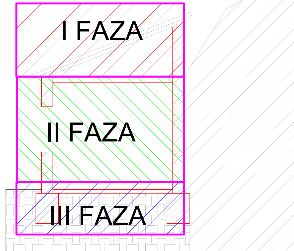
Presjek 1-1sa prikazanim fazama rušenja
