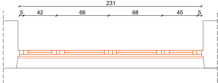
PR-08 OSNOVA
