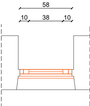
SU-06 OSNOVA
