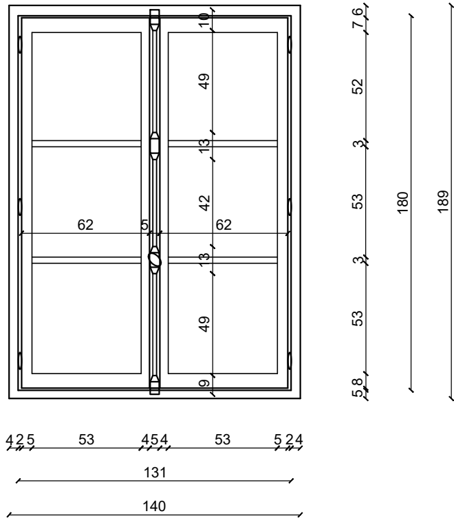
SU-07 PRESJEK
