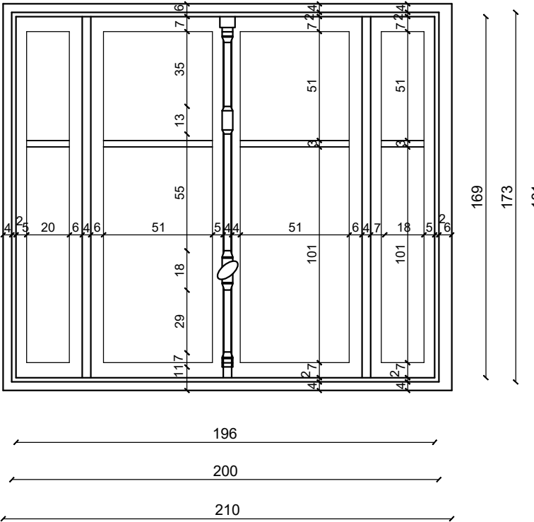
PK-05 OSNOVA
