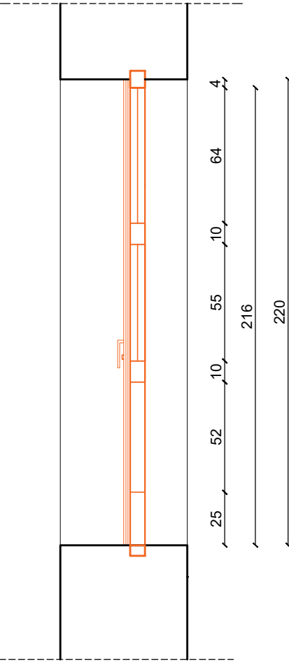
ST-02 PRESJEK
