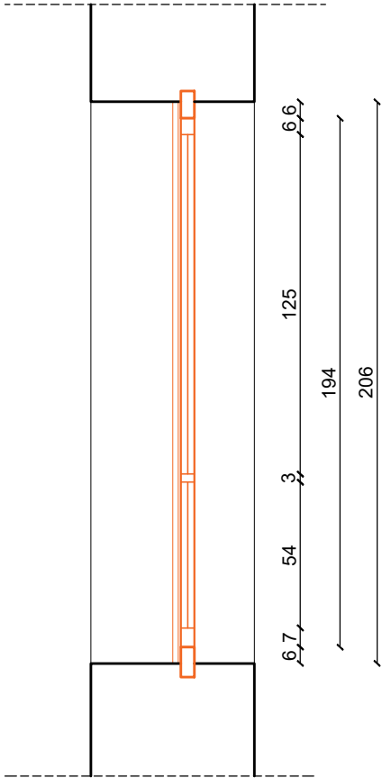
SP-08 PRESJEK
