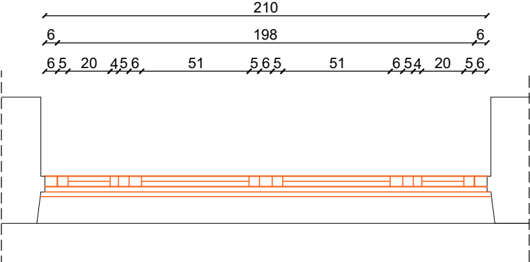
SP-19 OSNOVA
