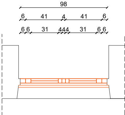
PK-07 OSNOVA
