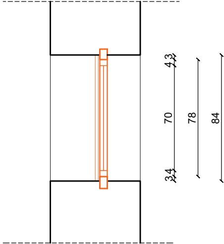
PK-02 PRESJEK
