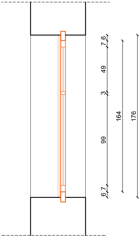
PK-12 PRESJEK
