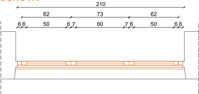
ST-03 OSNOVA
