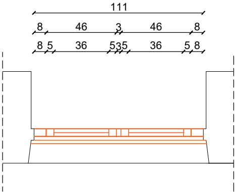
SP-09 OSNOVA
