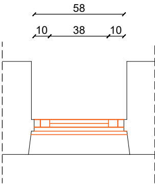
SU-06 OSNOVA
