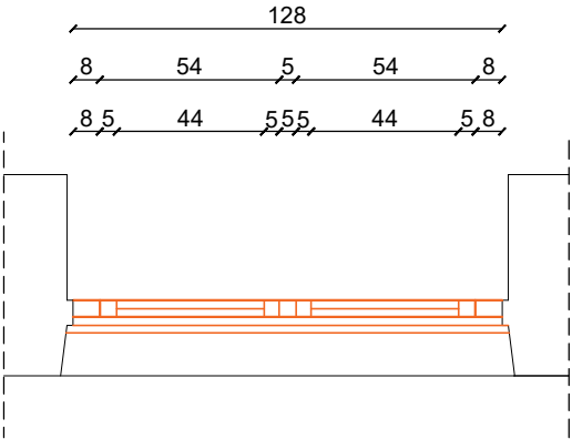
SP-12 OSNOVA
