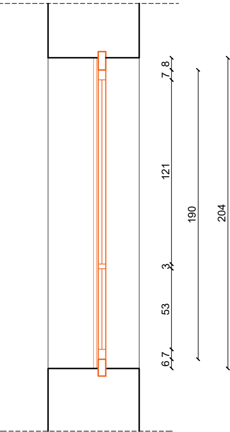
SP-03 PRESJEK
