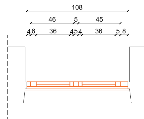
PK-04 OSNOVA
