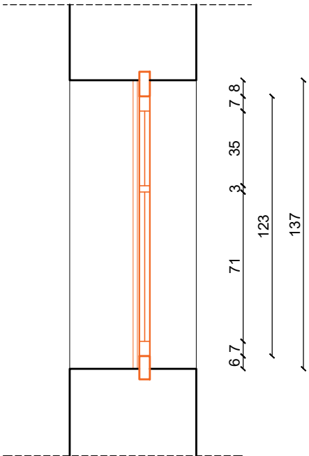
PK-04 PRESJEK
