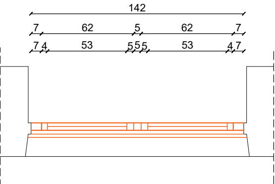
SP-16 OSNOVA
