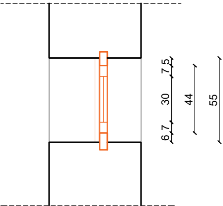
PK-08 PRESJEK
