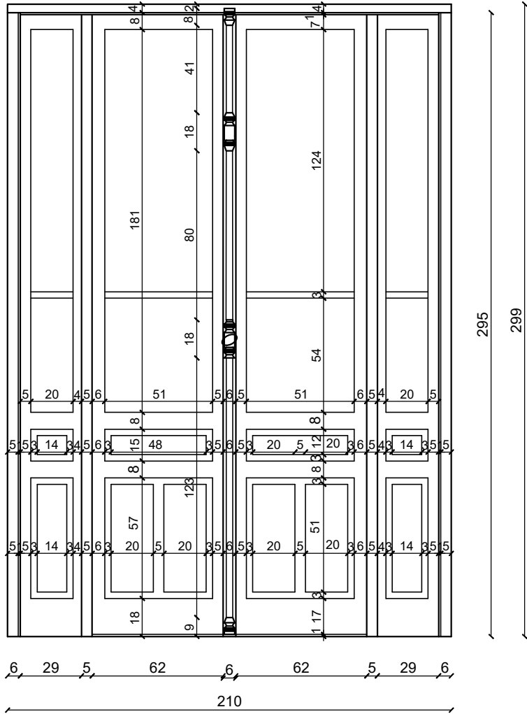
SP-10 OSNOVA
