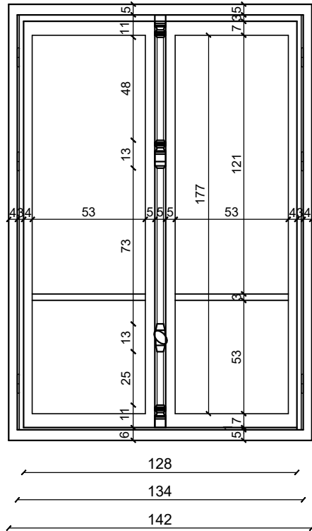
SP-01 OSNOVA
