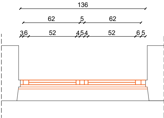
PK-03 OSNOVA
