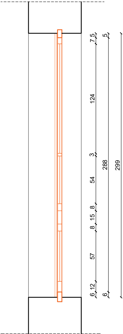
SP-19 PRESJEK
