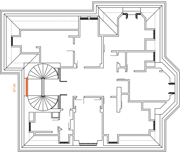
POTKROVLJE
