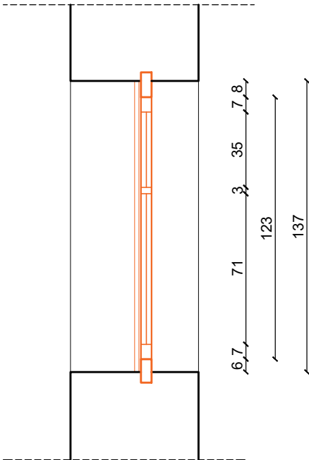
PK-04 PRESJEK
