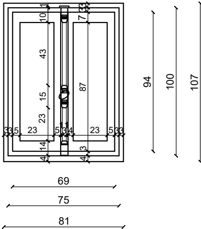
PK-11 OSNOVA
