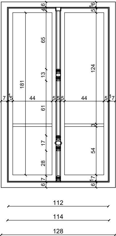
SP-12 OSNOVA
