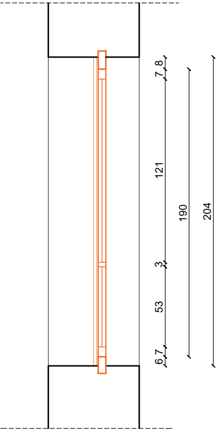
SP-01 PRESJEK
