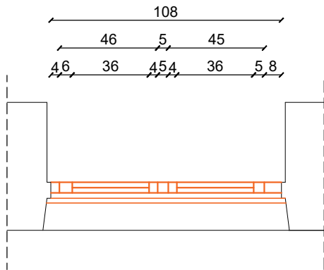
PK-04 OSNOVA
