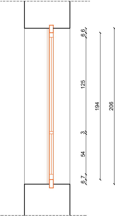
SP-09 PRESJEK
