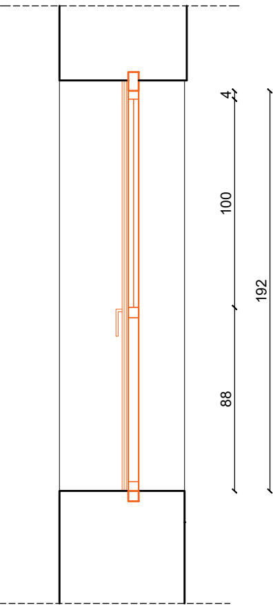
ST-01 PRESJEK
