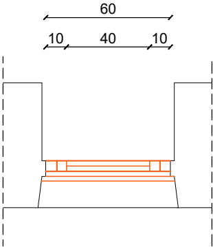
SU-02 OSNOVA
