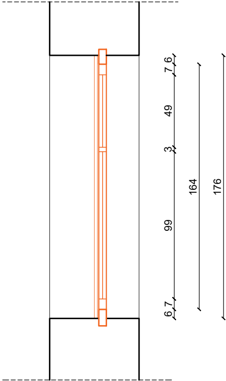
PK-12 PRESJEK
