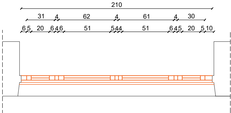
PK-05 OSNOVA
