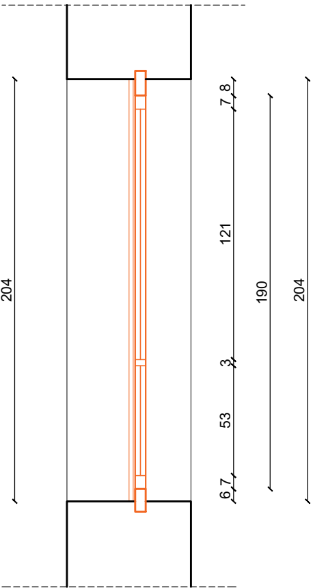
SP-02 PRESJEK
