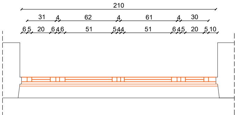
PK-05 OSNOVA
