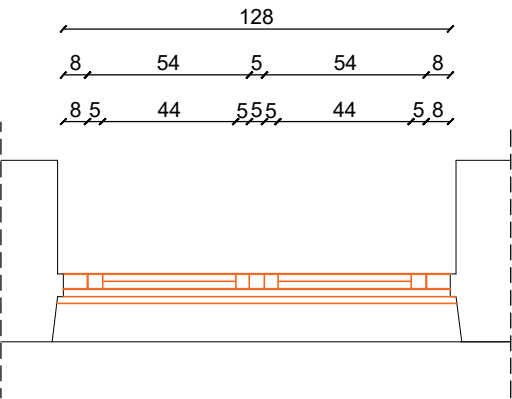
SP-07 OSNOVA
