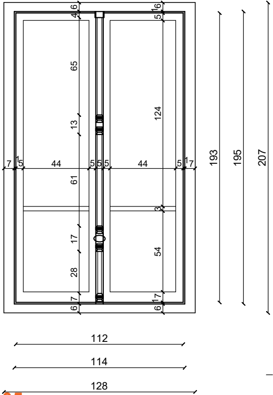
SP-05 OSNOVA
