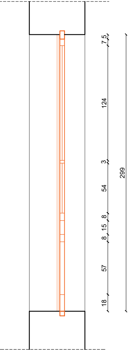
SP-10 PRESJEK
