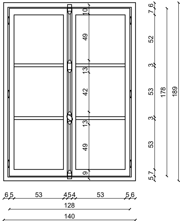
SU-08 OSNOVA
