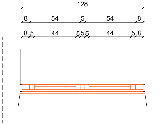
SP-06 OSNOVA
