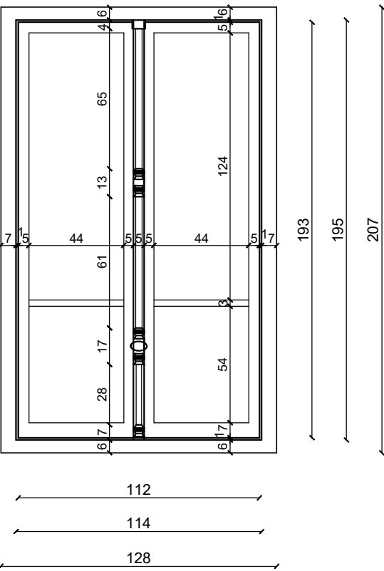
SP-07 OSNOVA
