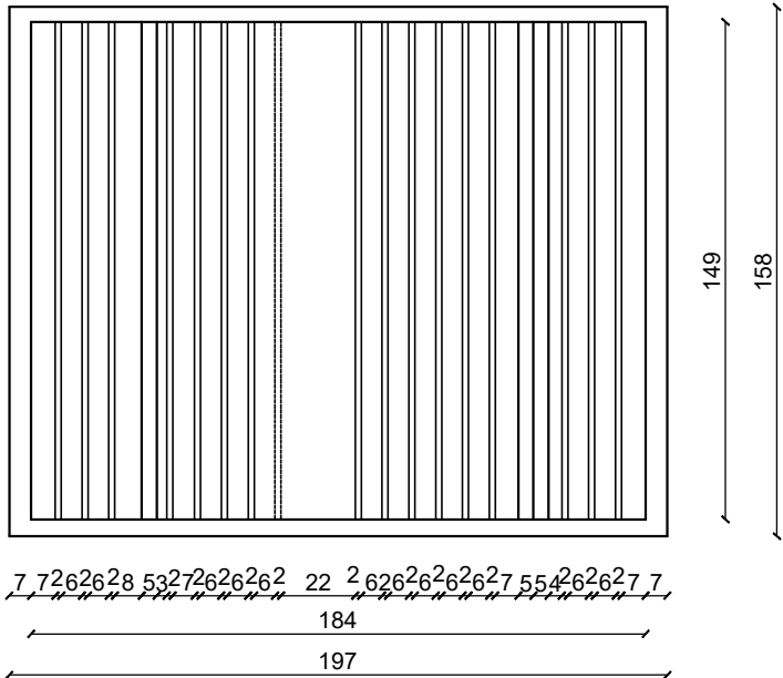
PK-06 OSNOVA
