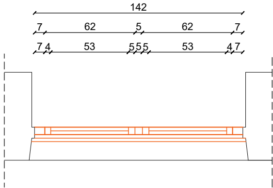
SP-01 OSNOVA
