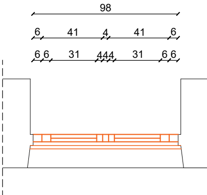
PK-10 OSNOVA
