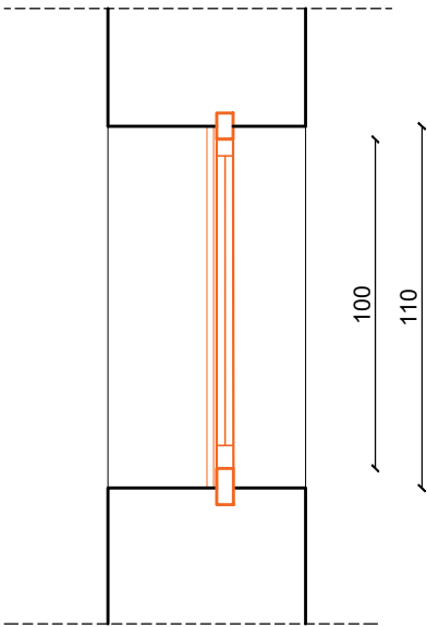
SU-05 PRESJEK
