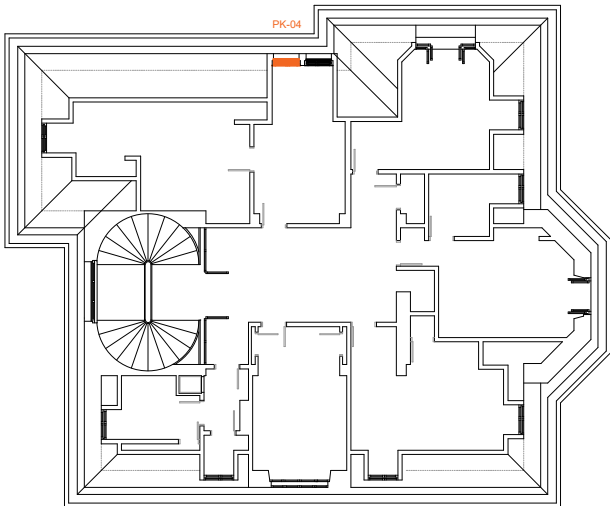
POTKROVLJE
