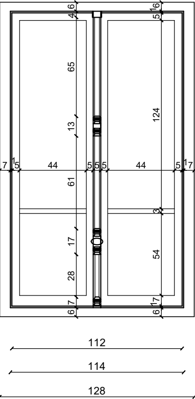
SP-06 OSNOVA
