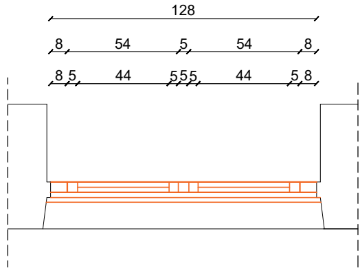
SP-04 OSNOVA
