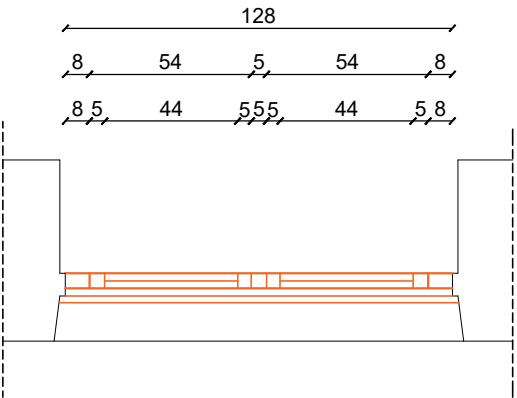
SP-11 OSNOVA
