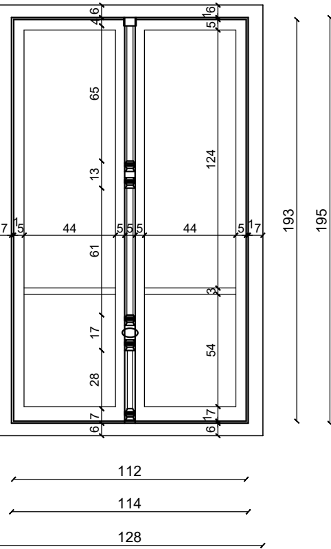
SP-04 OSNOVA
