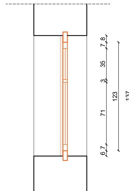
PK-04 PRESJEK
