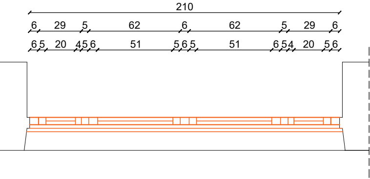
SP-10 OSNOVA
