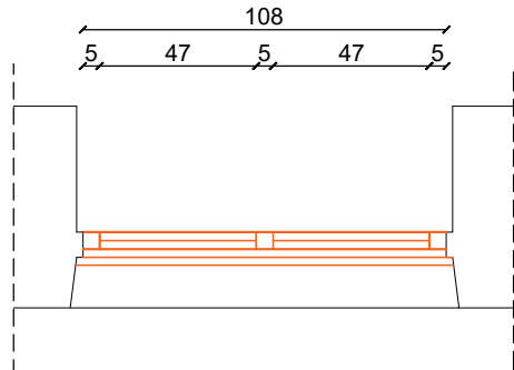
ST-01 OSNOVA
