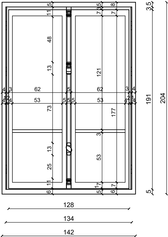
SP-17 OSNOVA
