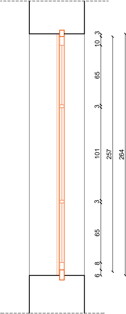
PR-10 PRESJEK
