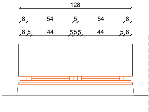
SP-04 OSNOVA
