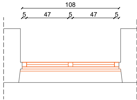
ST-01 OSNOVA
