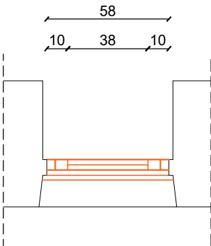
SU-04 OSNOVA
