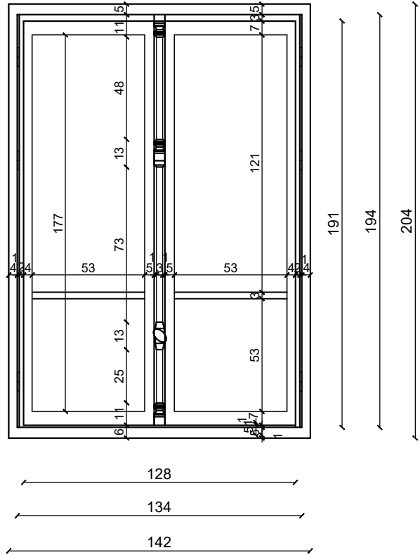
SP-03 OSNOVA
