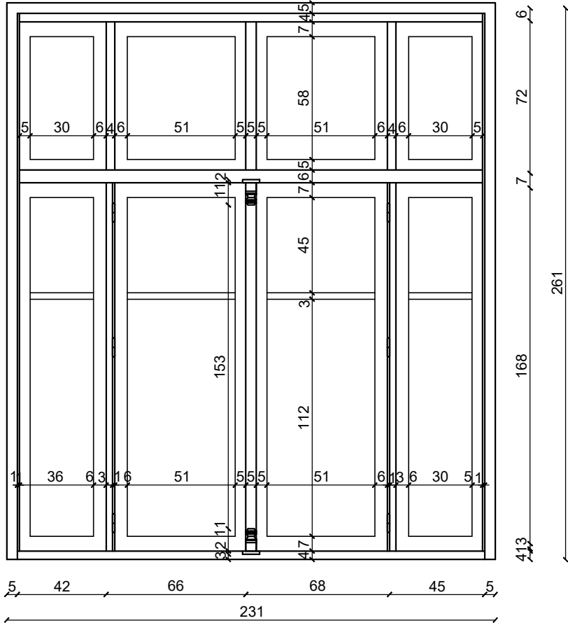
PR-08 OSNOVA
