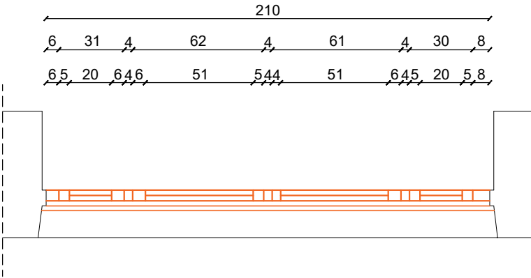
PK-12 OSNOVA
