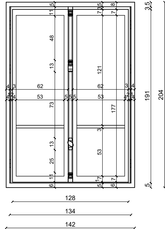
SP-18 OSNOVA
