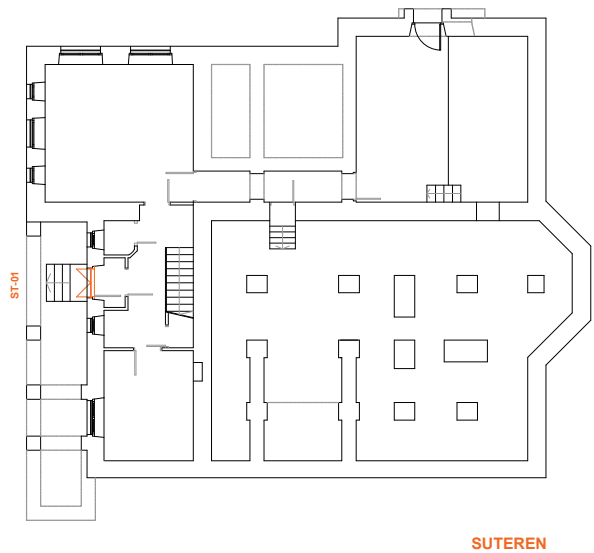
SUTEREN
