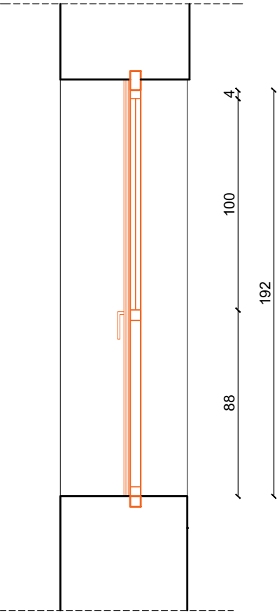
ST-01 PRESJEK
