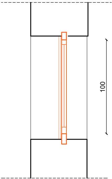
SU-01 PRESJEK
