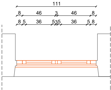
SP-09 OSNOVA
