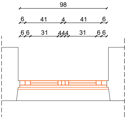
PK-10 OSNOVA
