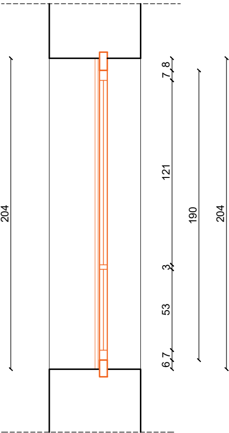
SP-02 PRESJEK
