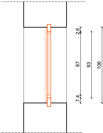
PK-01 PRESJEK
