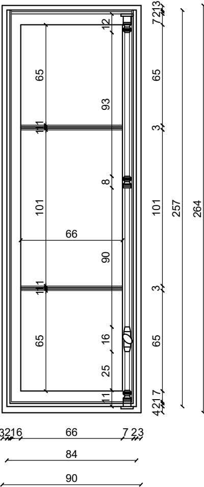
PR-10 OSNOVA
