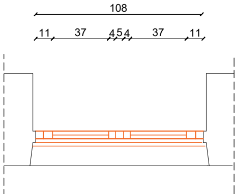
SU-05 OSNOVA
