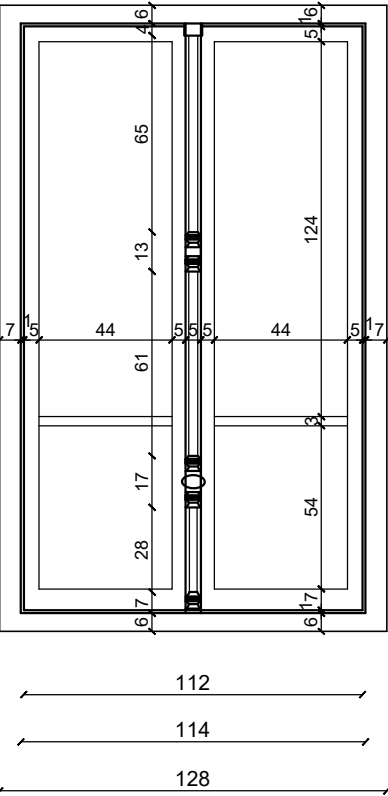
SP-04 OSNOVA
