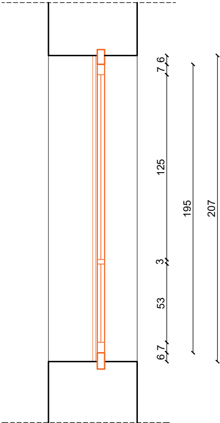
SP-13 PRESJEK
