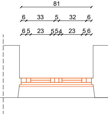
PK-11 OSNOVA
