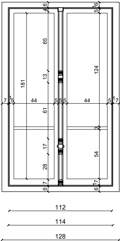
SP-11 OSNOVA
