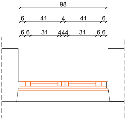
PK-08 OSNOVA
