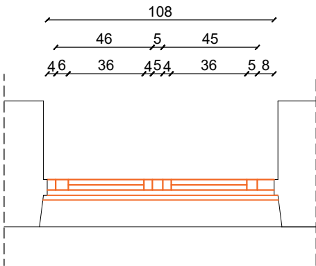
PK-04 OSNOVA
