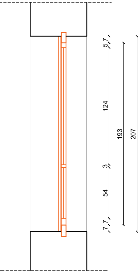
SP-07 PRESJEK
