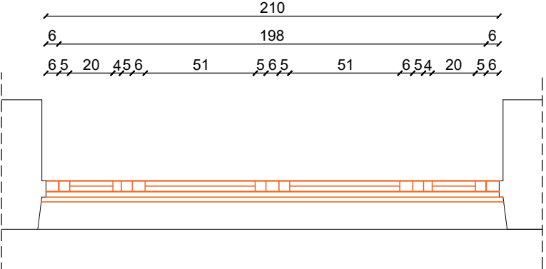
SP-19 OSNOVA
