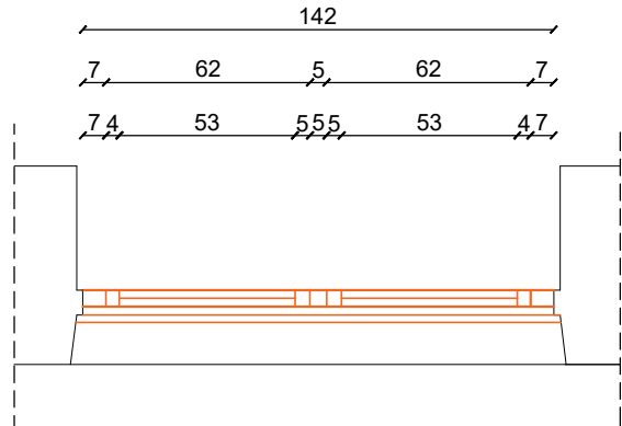
SP-03 OSNOVA
