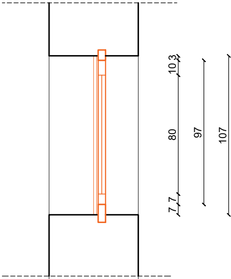
PK-11 PRESJEK
