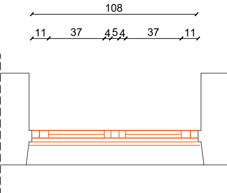
SU-05 OSNOVA
