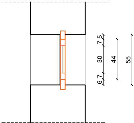
PK-08 PRESJEK
