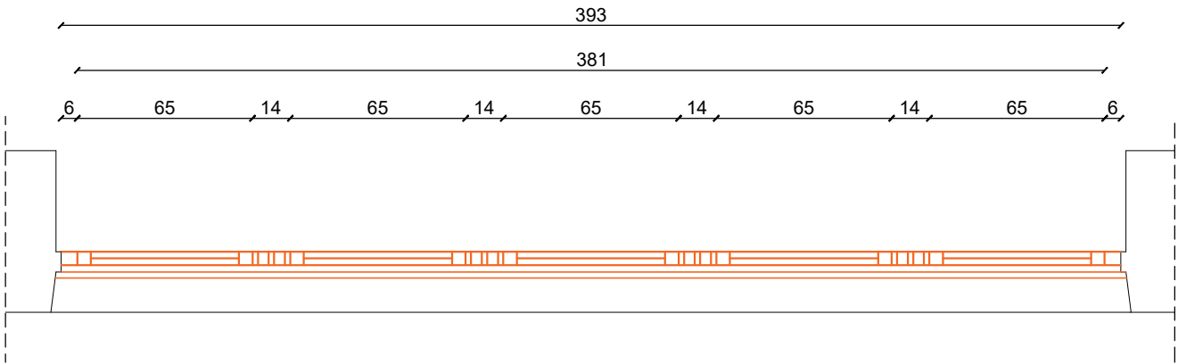
ST-04 OSNOVA
