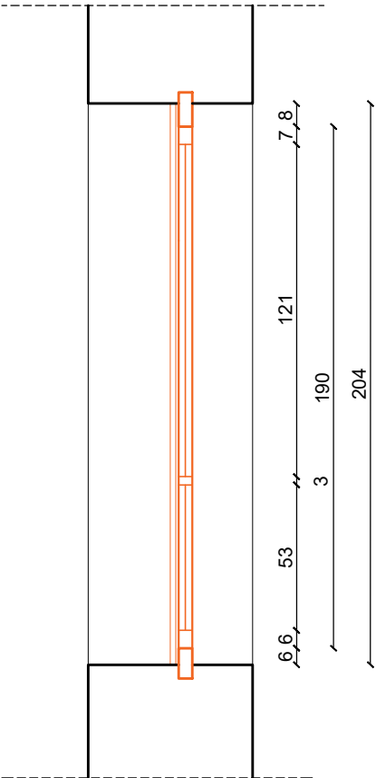
SP-16 PRESJEK
