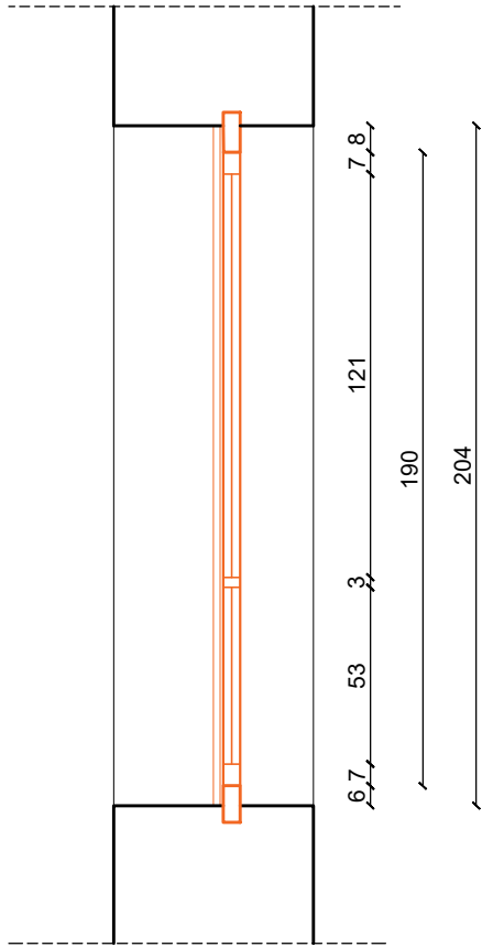
SP-01 PRESJEK
