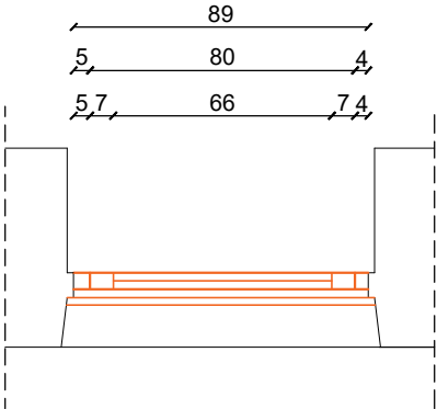
SP-13 OSNOVA
