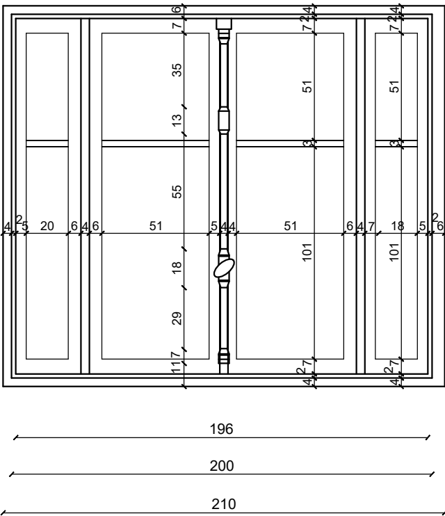
PK-05 OSNOVA
