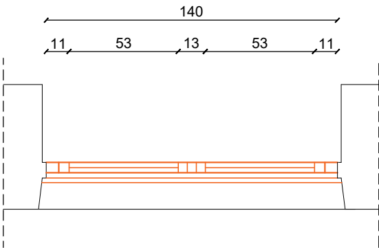
SU-07 PRESJEK
