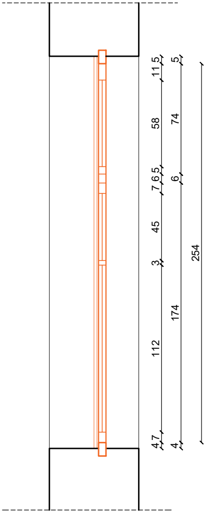
PR-08 PRESJEK
