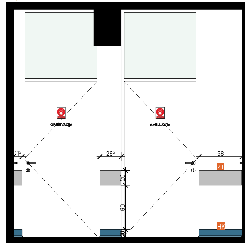
IZGLED 4
