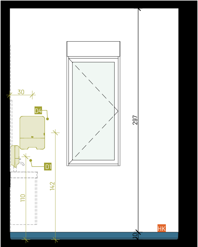
IZGLED 10
