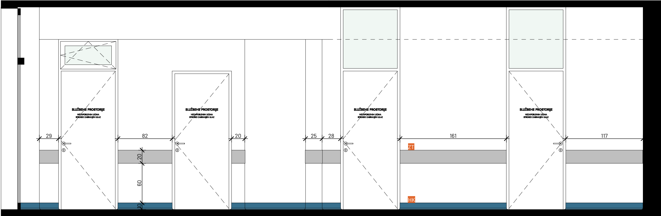
IZGLED 1
