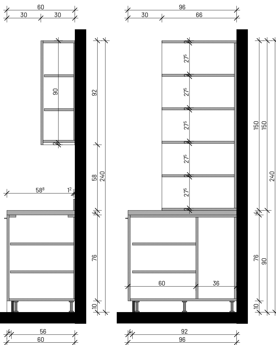
Presjek B-B
