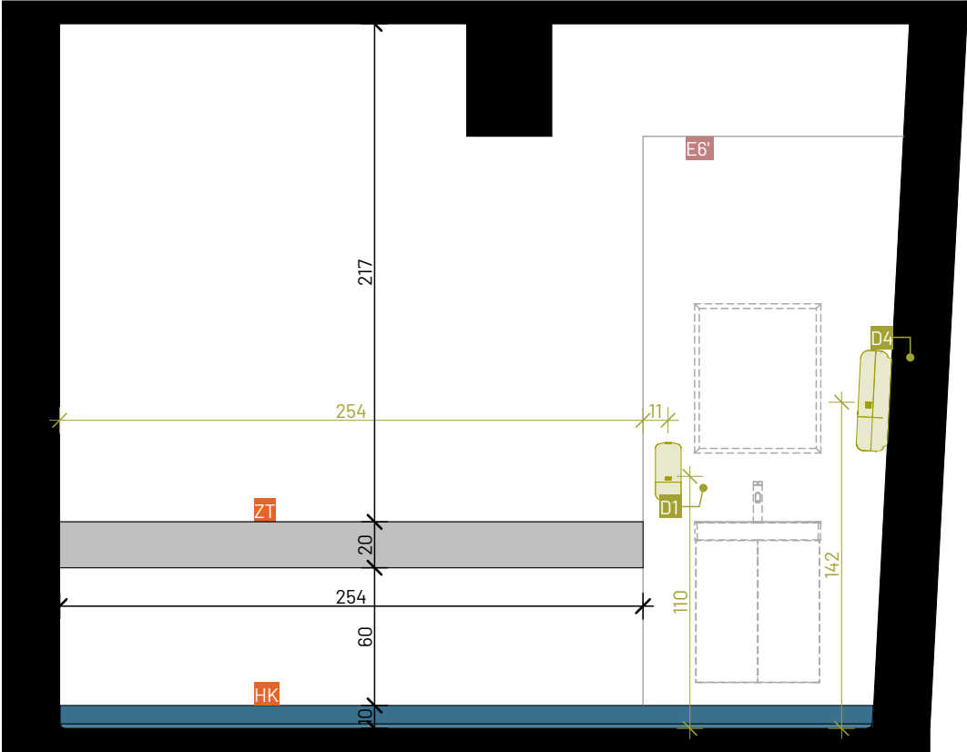
IZGLED 9
