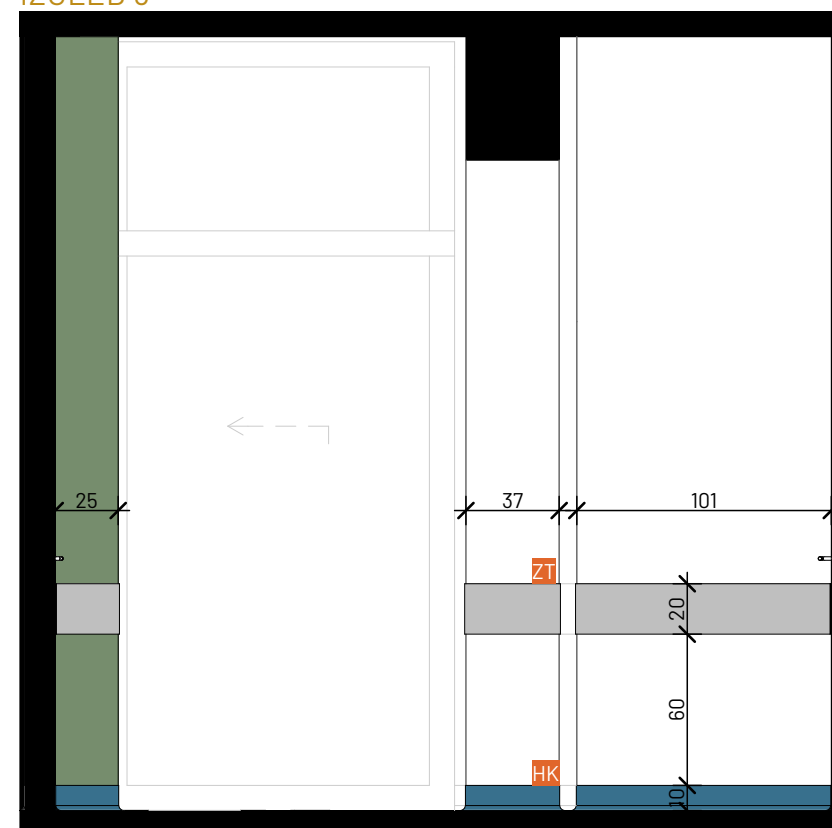
IZGLED 6
