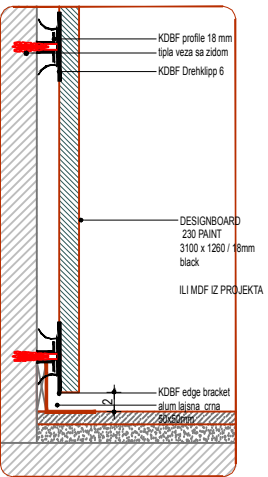
Detalj A
