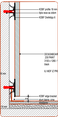
Detalj A
