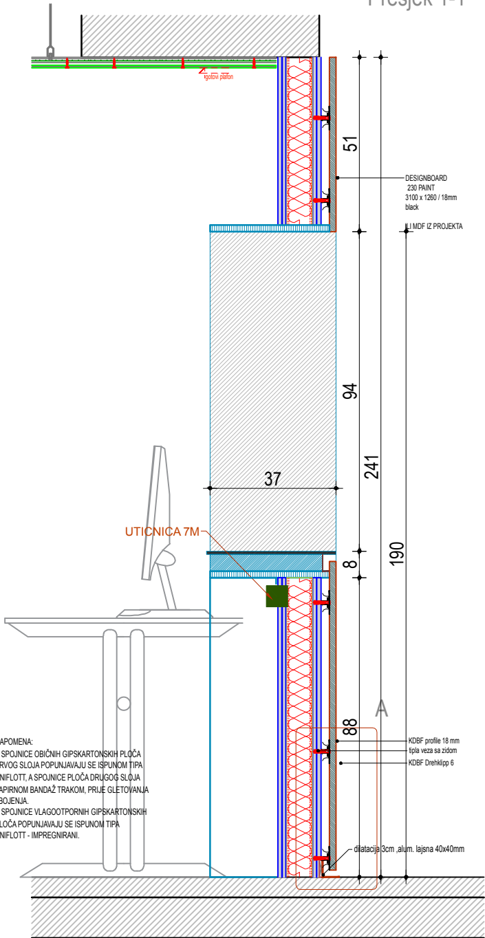
Presjek 1-1
