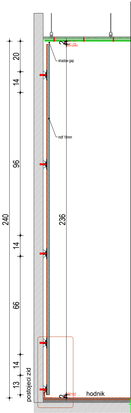
Presjek 1-1
