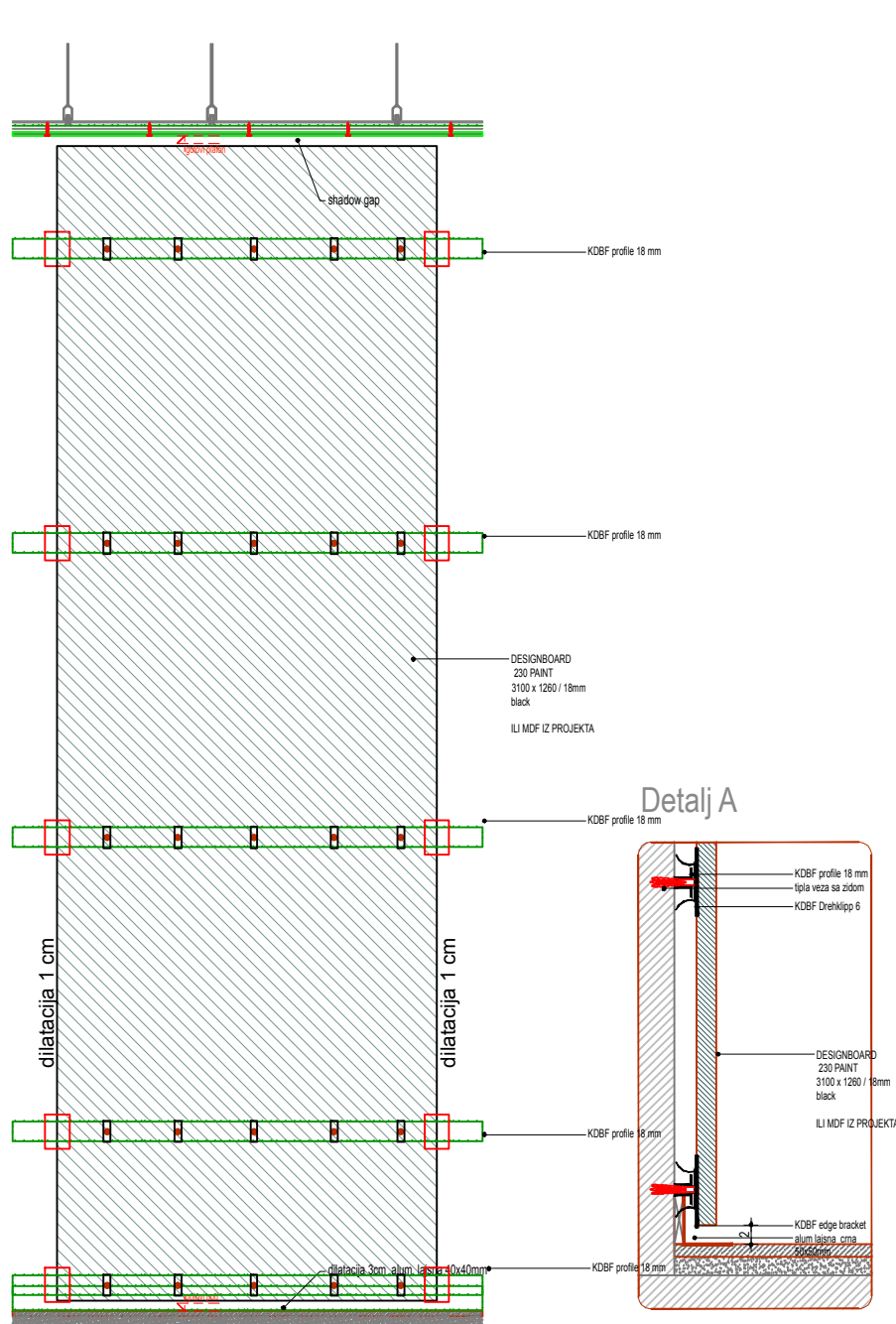
Izgled 1-1
