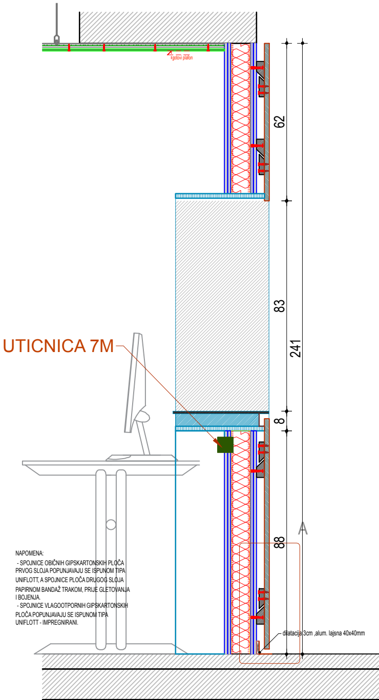
Presjek 1-1
