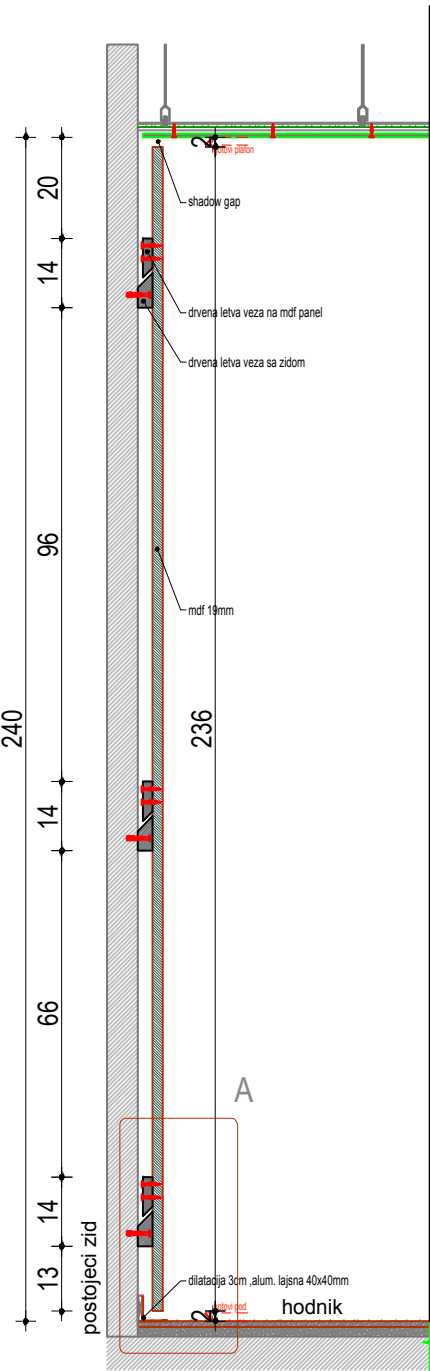
Presjek 1-1
