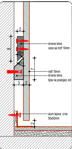
Detalj A
